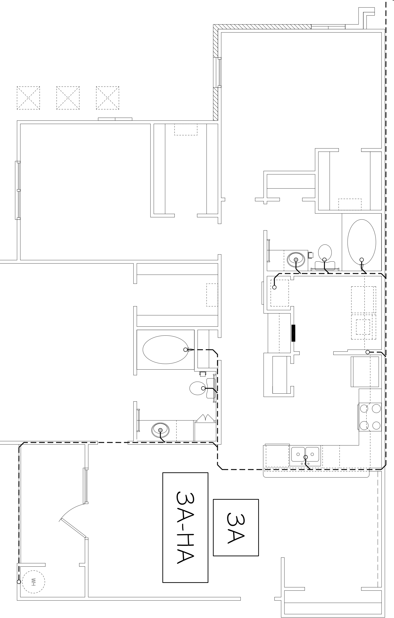
UNIT 3A SEWER PLUMBING RISER SCALE: 1/4" = 1'-0"
