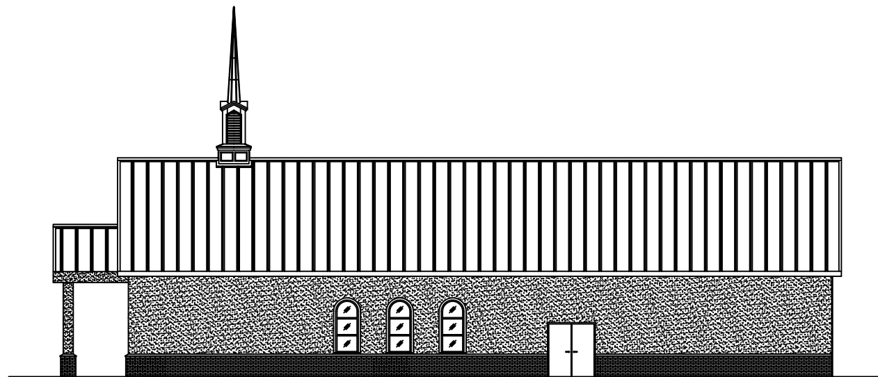
RIGHT ELEVATION SCALE: 1/8"=1'
