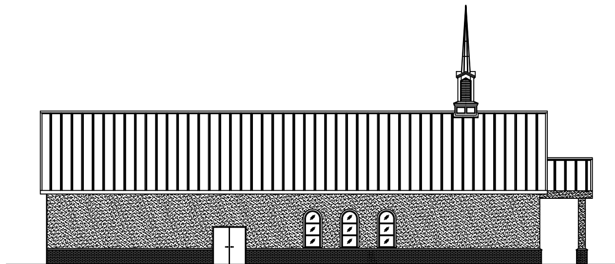
LEFT ELEVATION SCALE: 1/8"=1'
