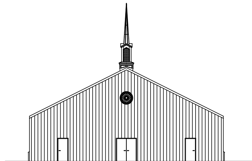
REAR ELEVATION SCALE: 1/8"=1'
