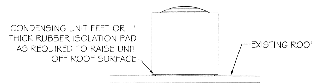
CONDENSING MOUNTING DETAIL N.T.S.
