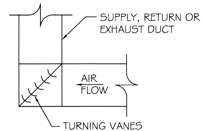
SQUARE ELBOW DETAIL N.T.S.
