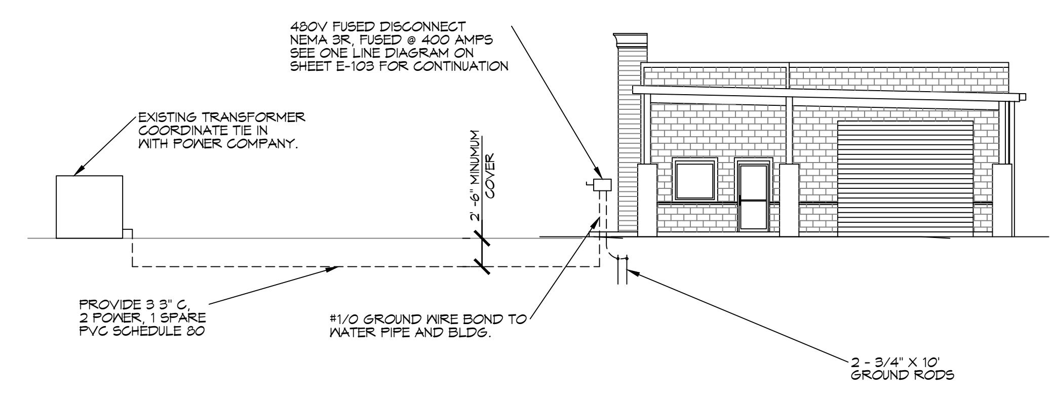
18 RISER DIAGRAM SCALE: N. T. S.
