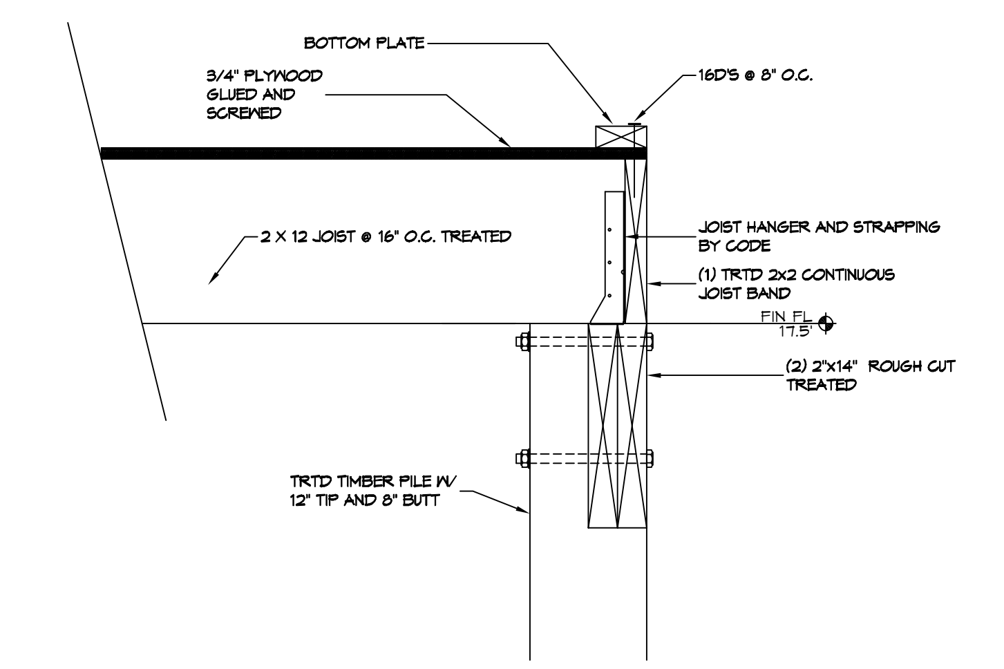
DETAIL SCALE: 1-1/2" = 1'-0"
