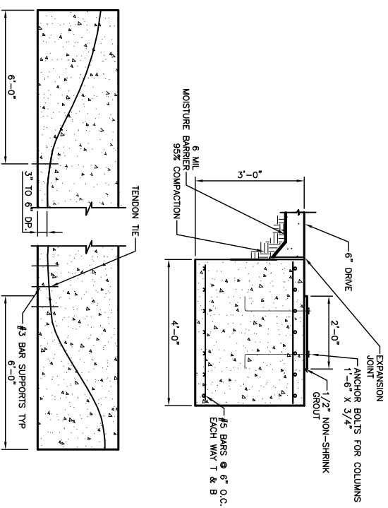
TYPICAL BEAM N.T.S.
