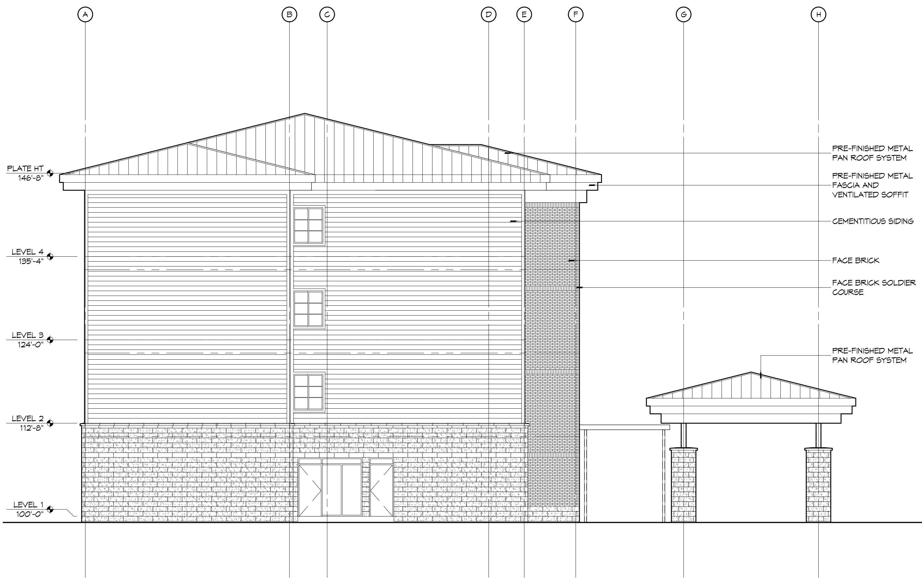
3 EXTERIOR ELEVATION SCALE: 1/8" = 1'-0"
