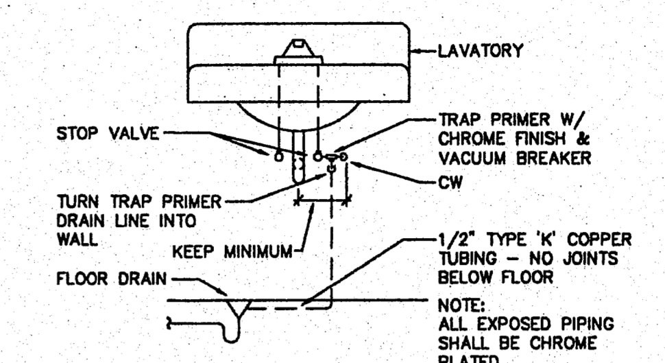
TRAP PRIMER DETAIL NOT TO SCALE
