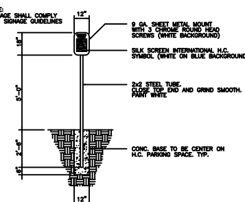
EXTERIOR HANDICAP SIGN N.T.S.
