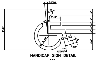
HANDICAP SIGN DETAIL N.T.S.
