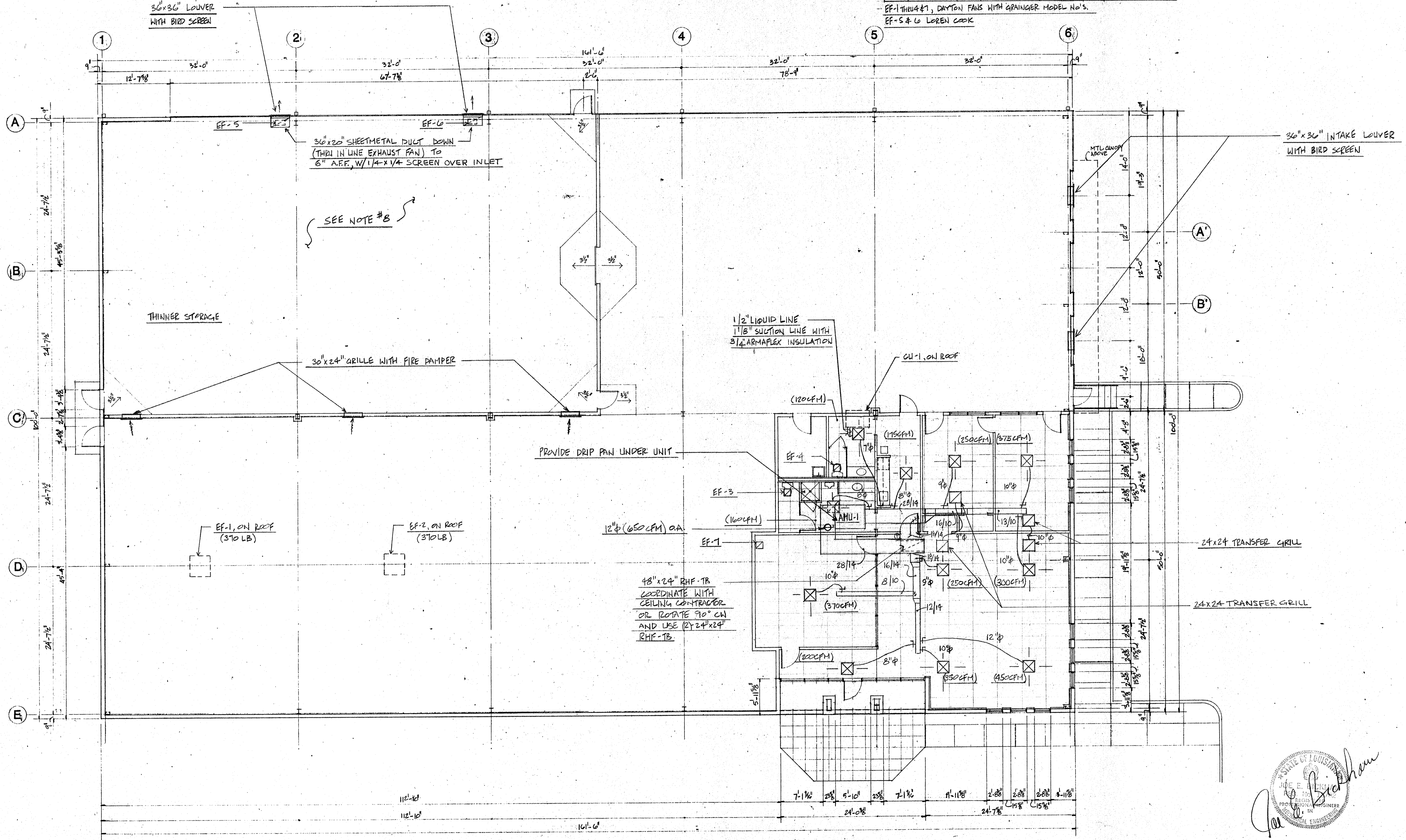
hvac plan scale: 1/8"=1'-0"
