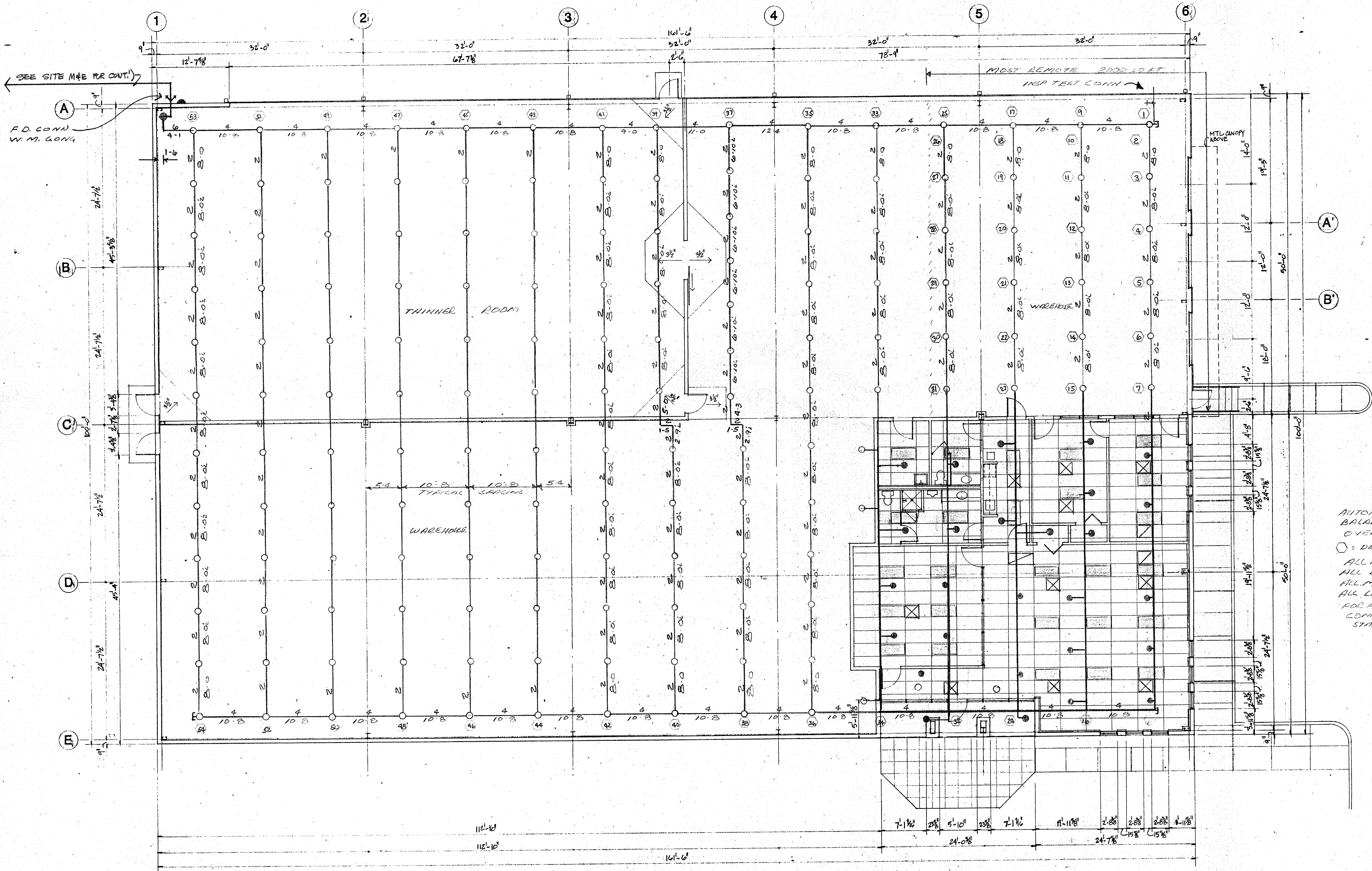
sprinkler plan scale: 1/8" = 1'-0"
