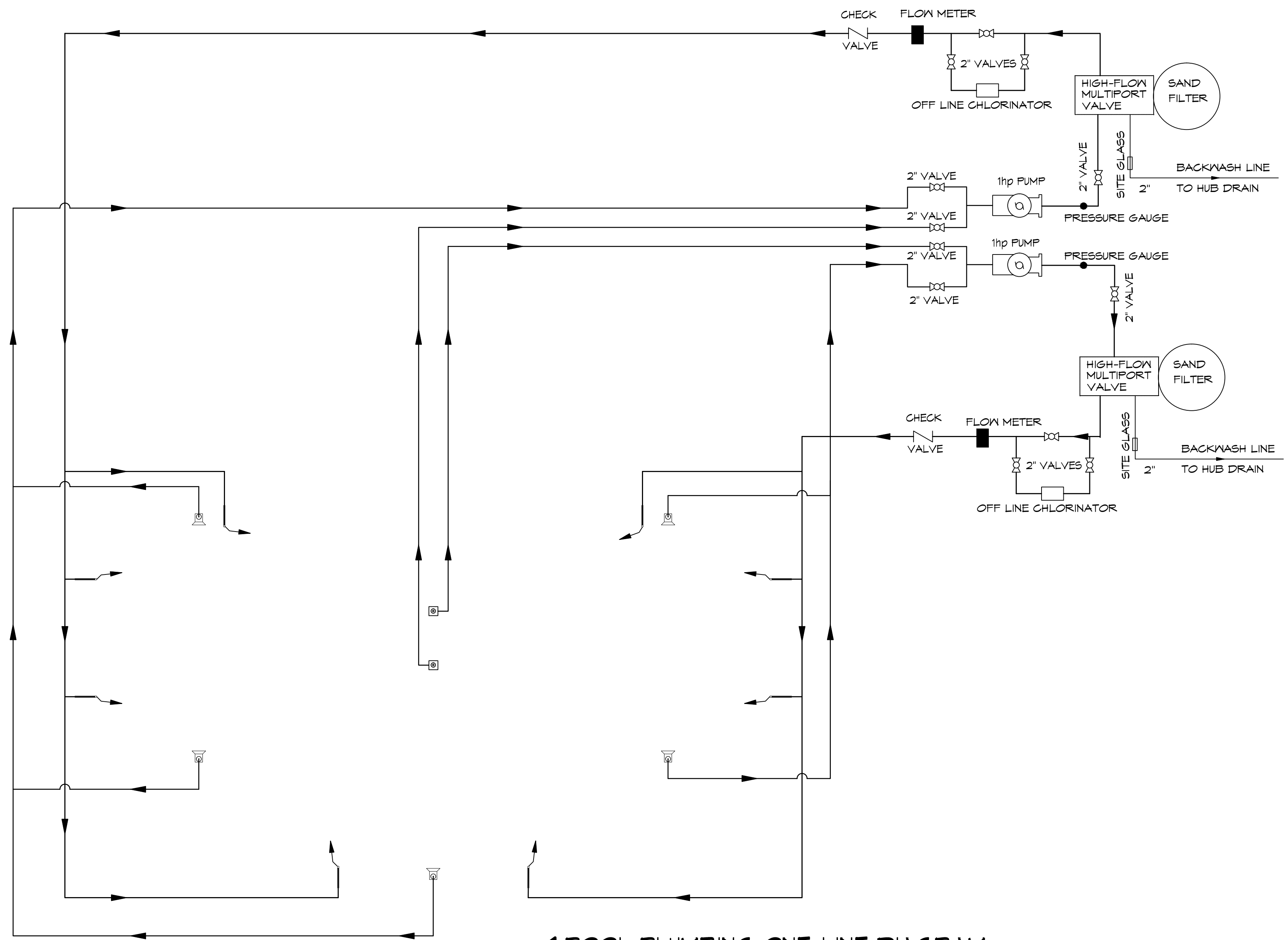
1 POOL PLUMBING ONE-LINE DIAGRAM SCALE: N.T.S.
