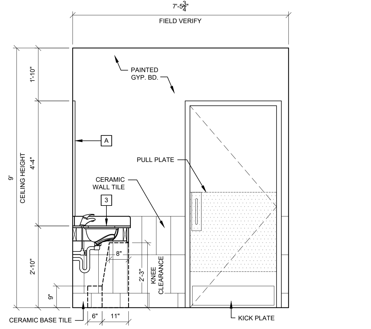
4 ELEVATION SCALE: 1/2" = 1'-0"
