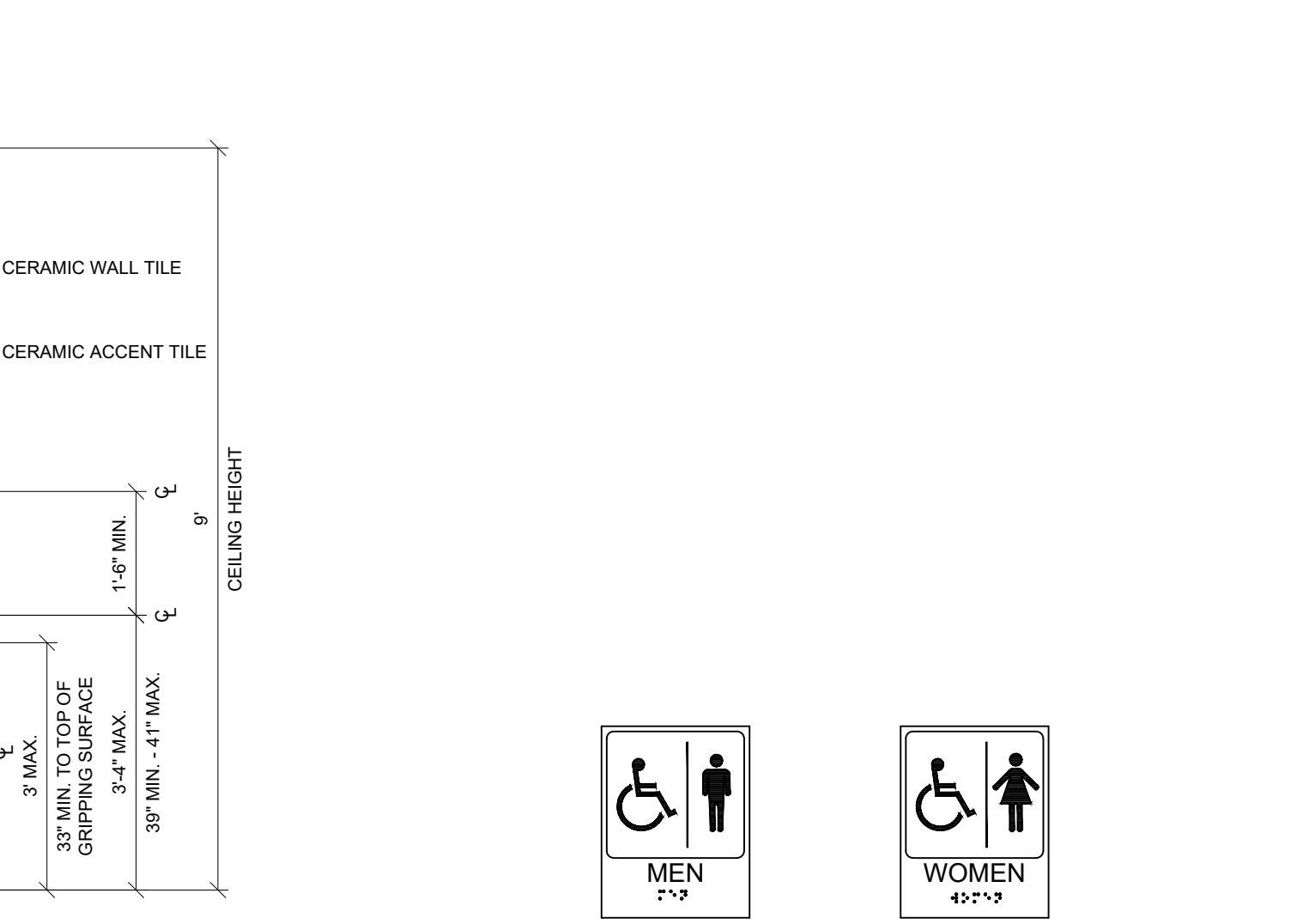
11 ELEVATION - VESTIBULE SCALE: 1/2" = 1'-0"
