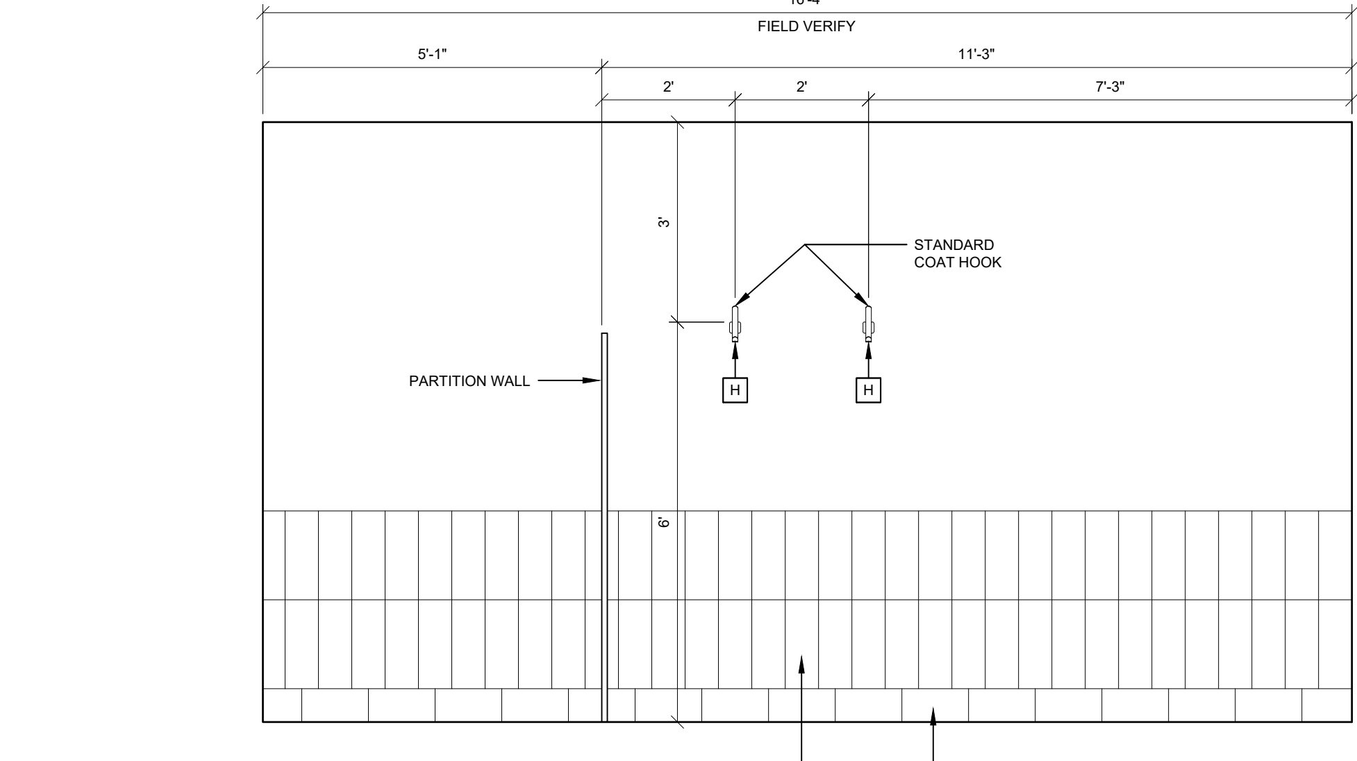
9 ELEVATION SCALE: 1/2" = 1'-0"
