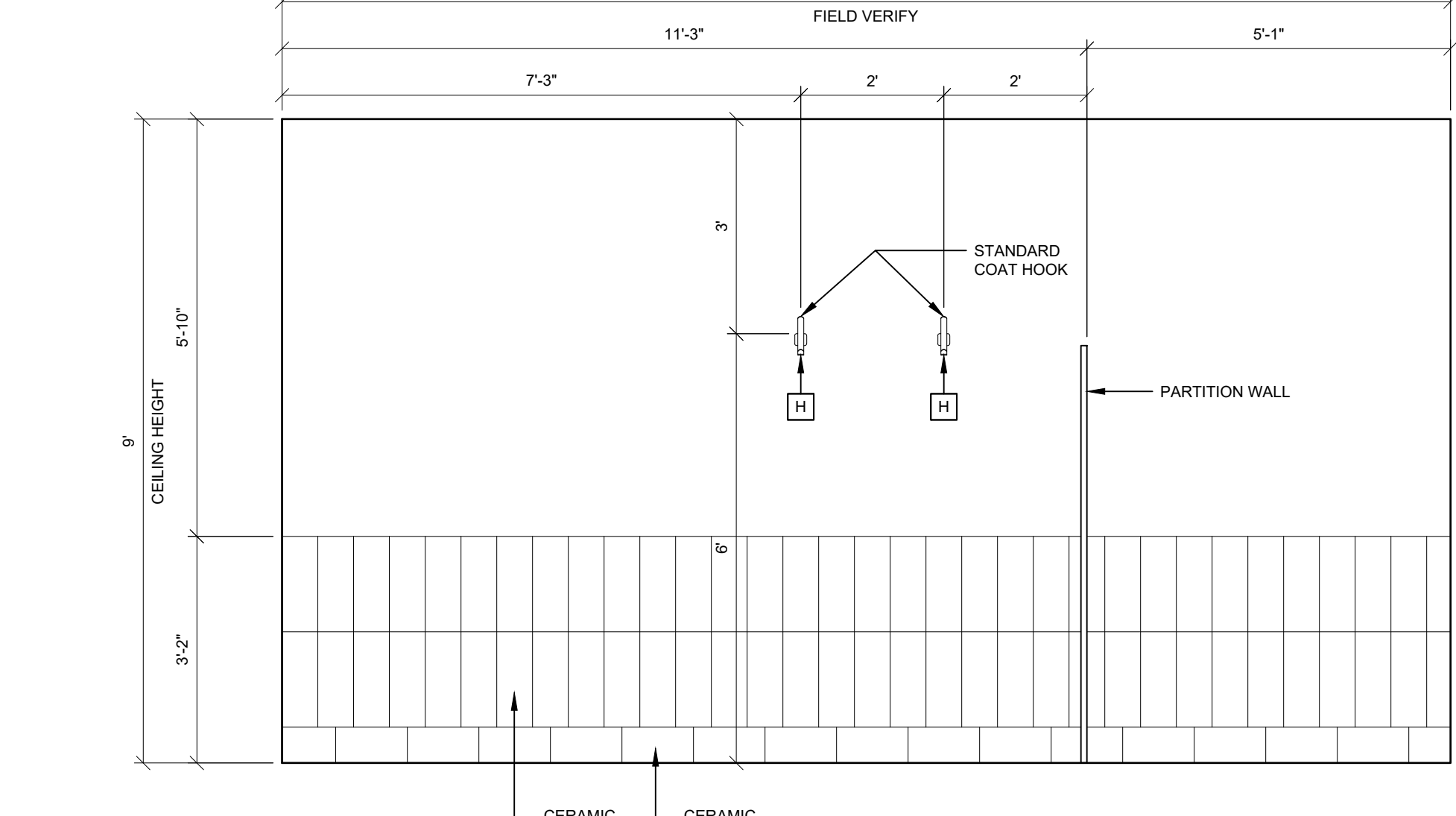
5 ELEVATION SCALE: 1/2" = 1'-0"
