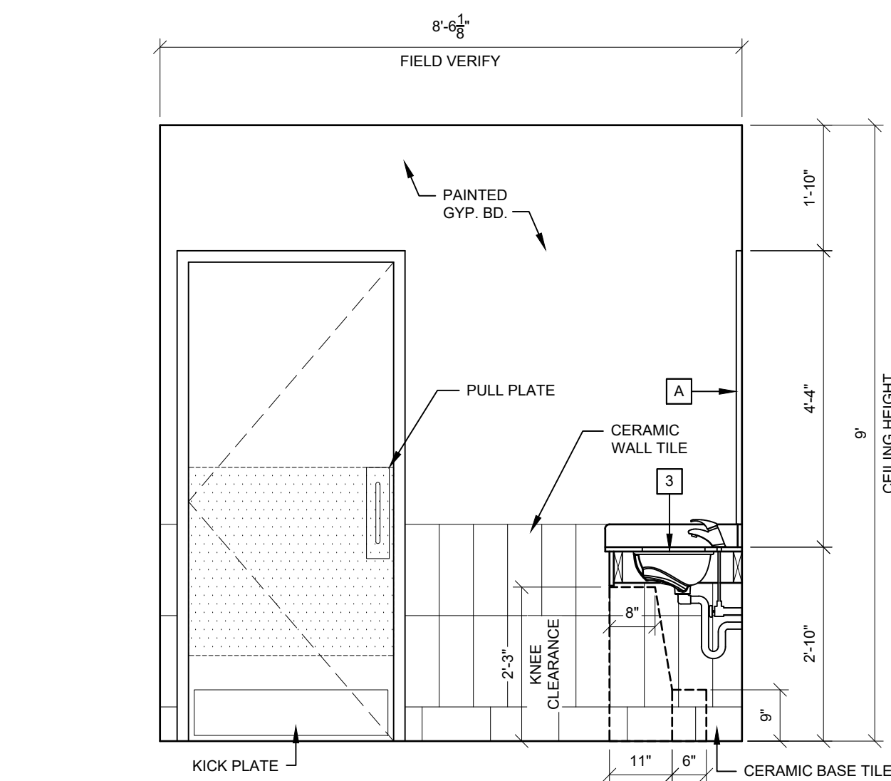
8 ELEVATION SCALE: 1/2" = 1'-0"
