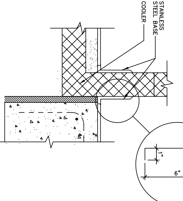
1B BASE DETAIL SCALE: 1 1/2" = 1'-0"
