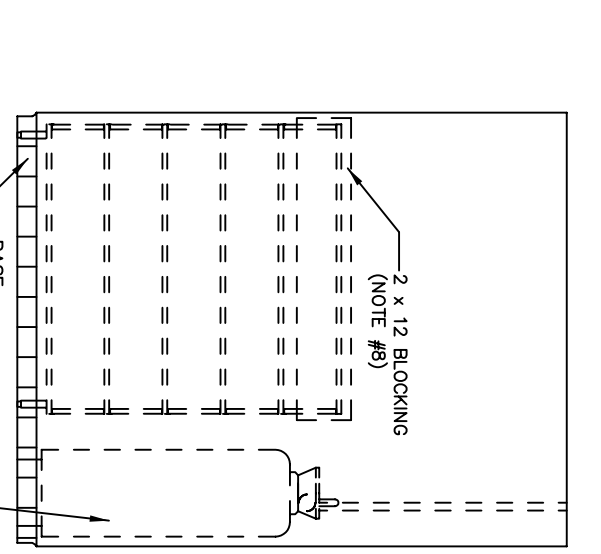
65 DRY STORAGE SCALE: 3/8" = 1'-0"
