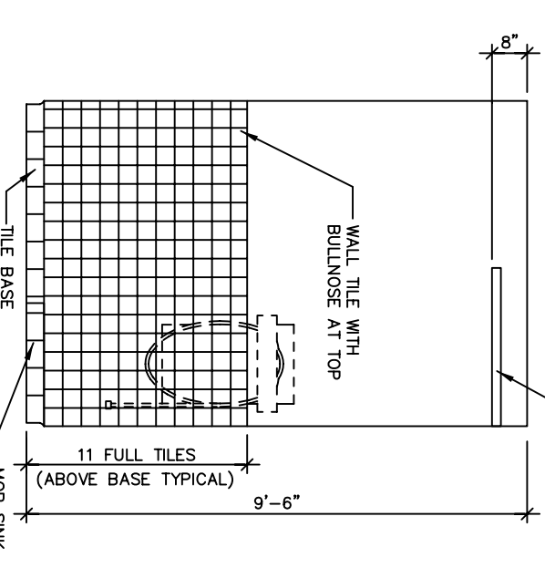
53 CHEM. ROOM SCALE: 3/8" = 1'-0"
