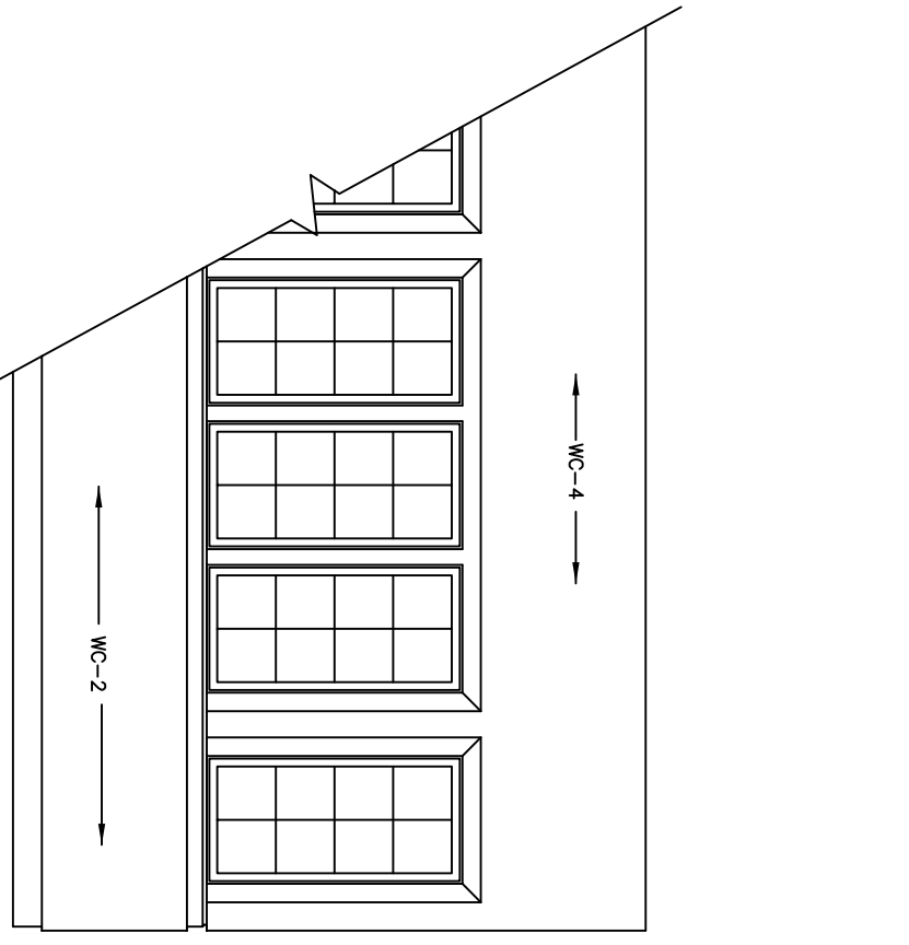
57A DINING AREA SCALE: 3/8" = 1'-0"
