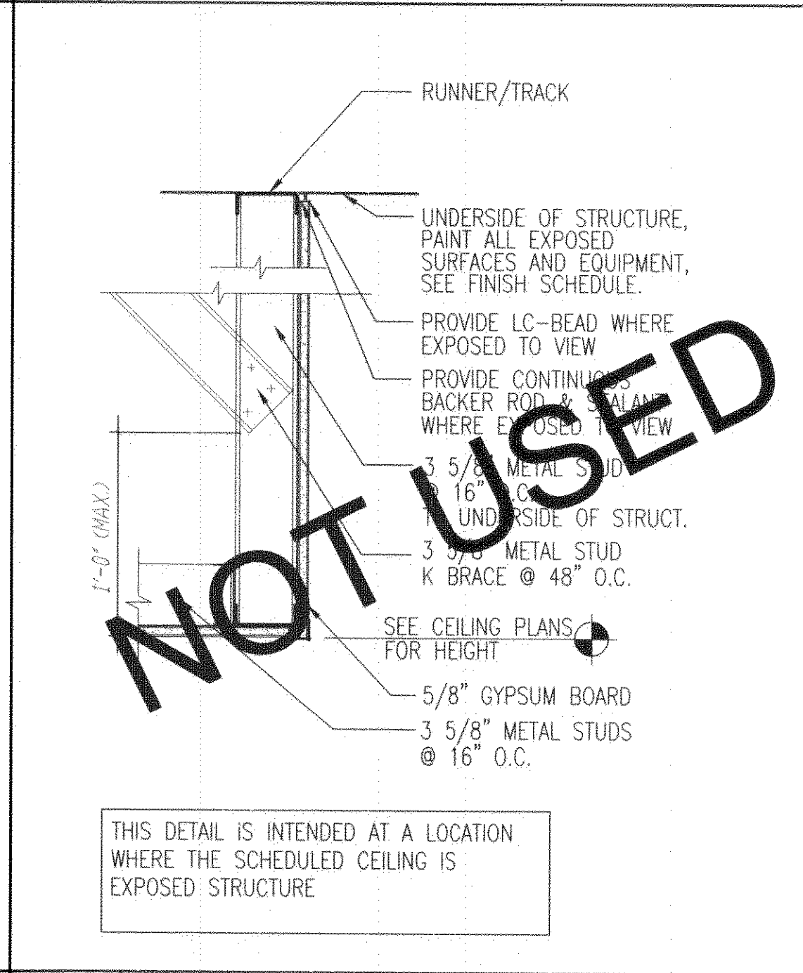
10 FASCIA/SOFFIT
