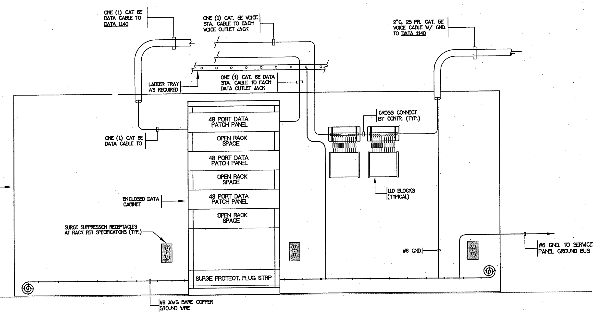
TYP. DATA ROOM (1203, 1213, 2201, 2217 & 2225)
