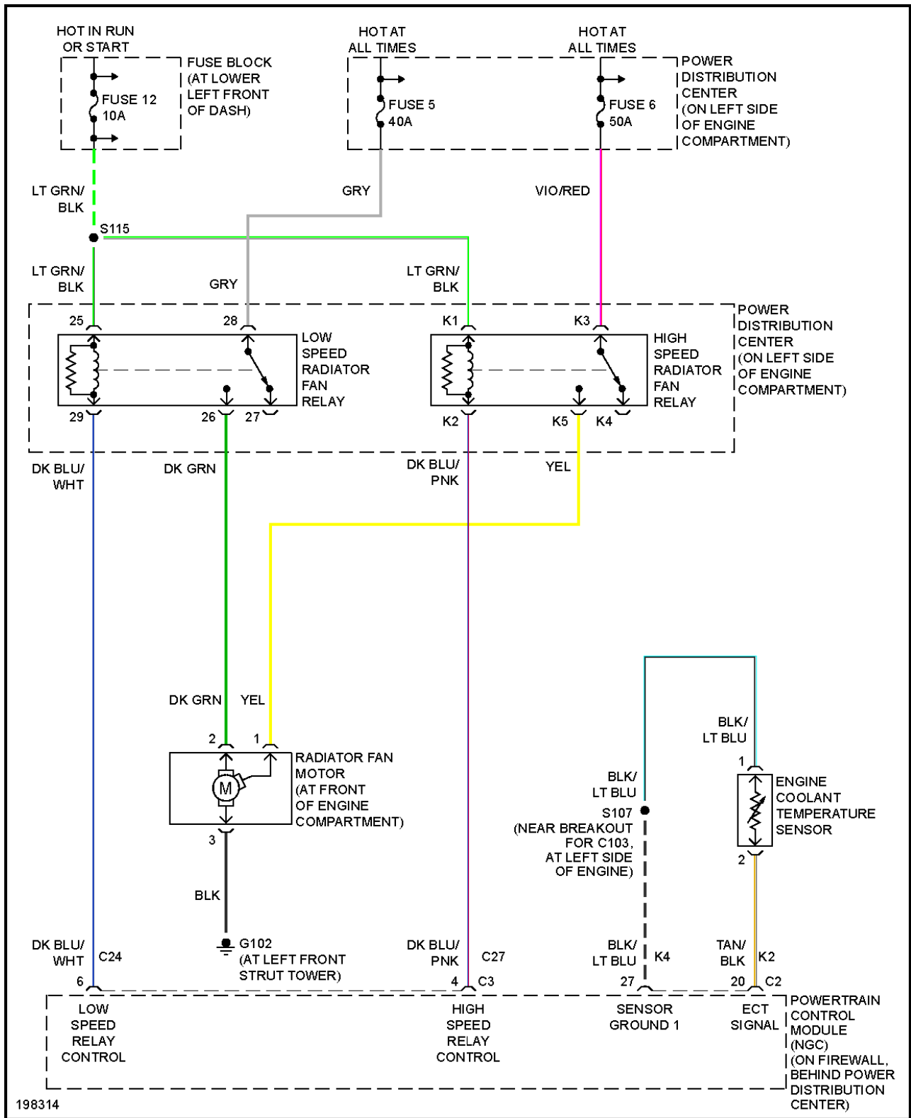
Fig. 8: 2.4L Turbo, Cooling Fan Circuit
