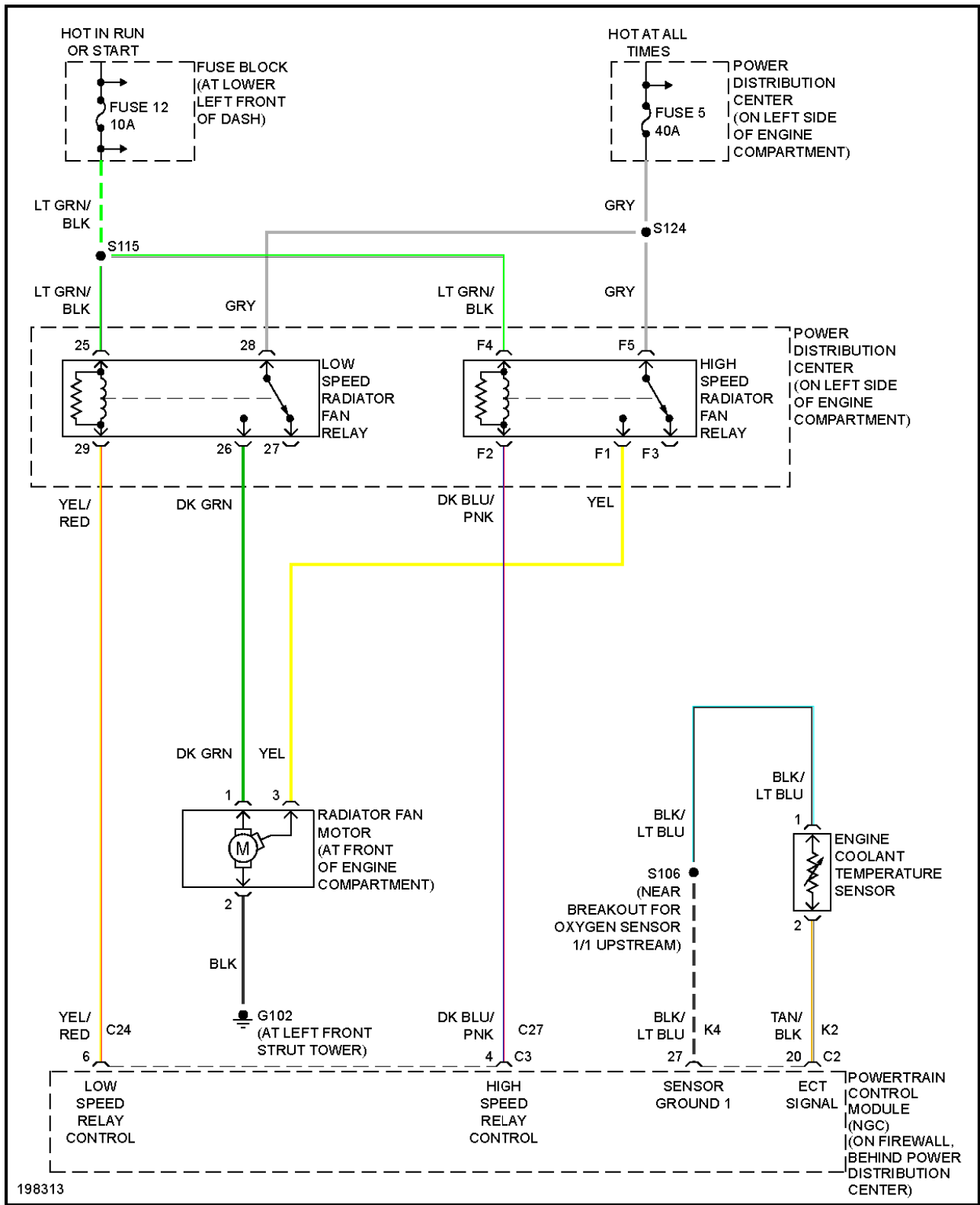
Fig. 7: 2.4L, Cooling Fan Circuit
