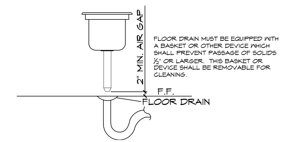
FLOOR SINK DRAIN SCALE: N.T.S.
