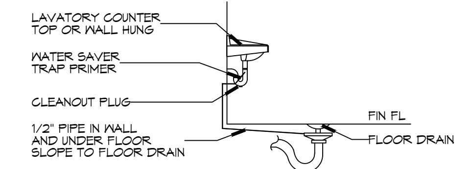
15 FLOOR DRAIN SCALE: N.T.S.
