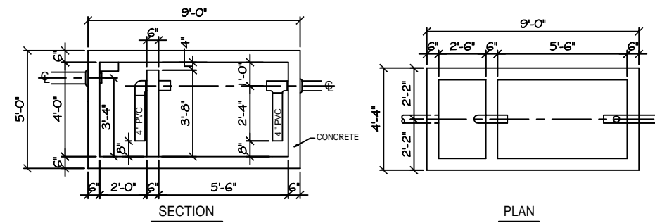
OIL/WATER SEPARATOR N.T.S.
