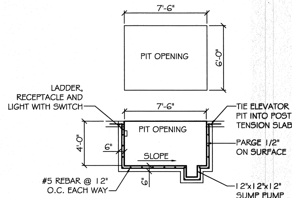
ELEVATOR PIT DETAIL SCALE: N.T.S.
