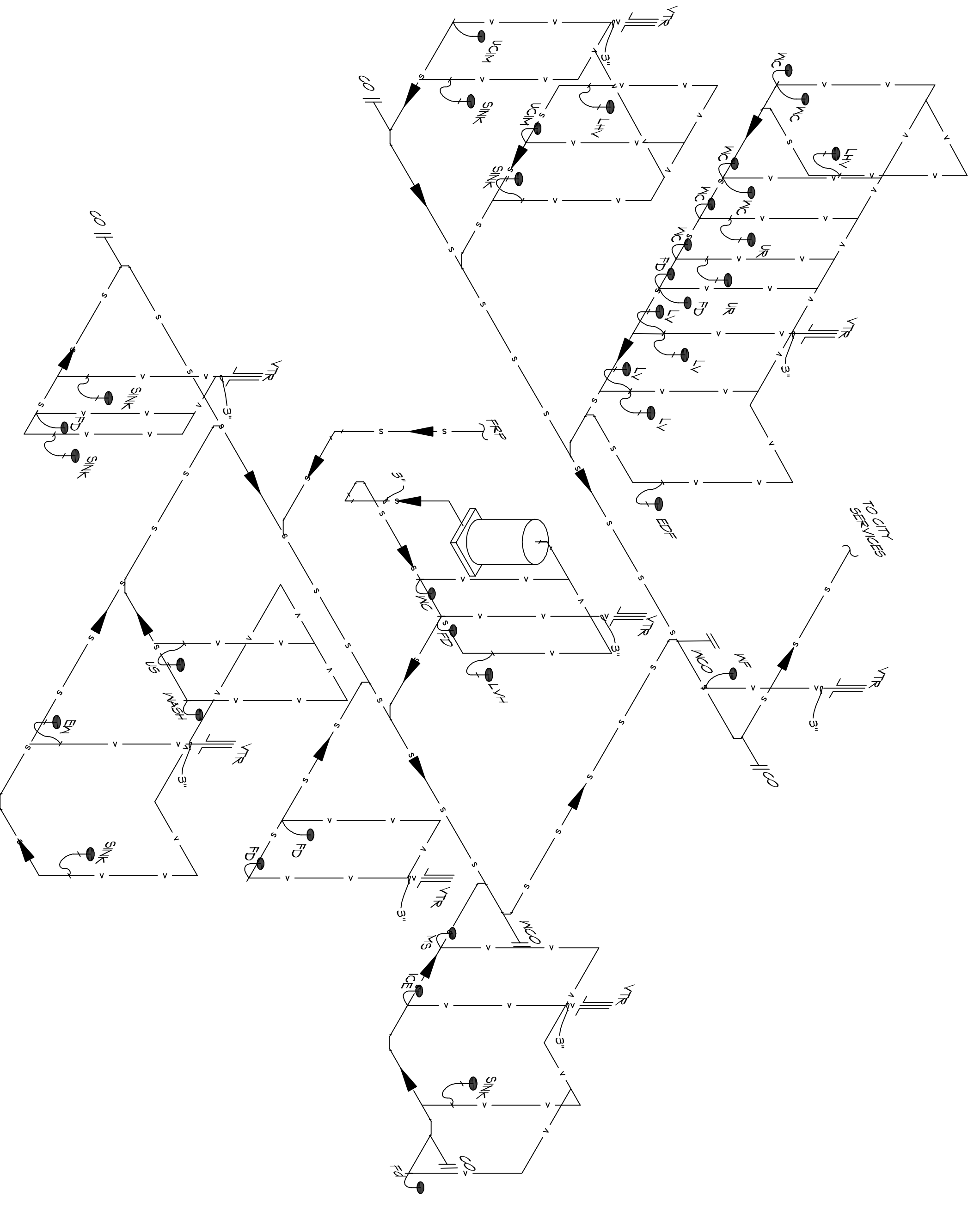
1 PLUMBING FIRST FLOOR RISER DIAGRAM SCALE: N.T.S.
