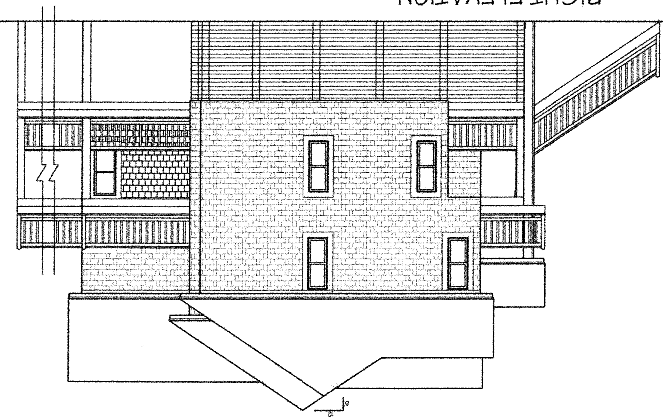
RIGHT ELEVATION
