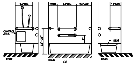
FIG. 32 TOILET STALL CLEARANCES N.T.S.
