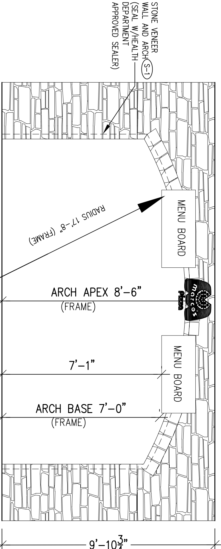
SCALE: 3/8" = 1'-0"
