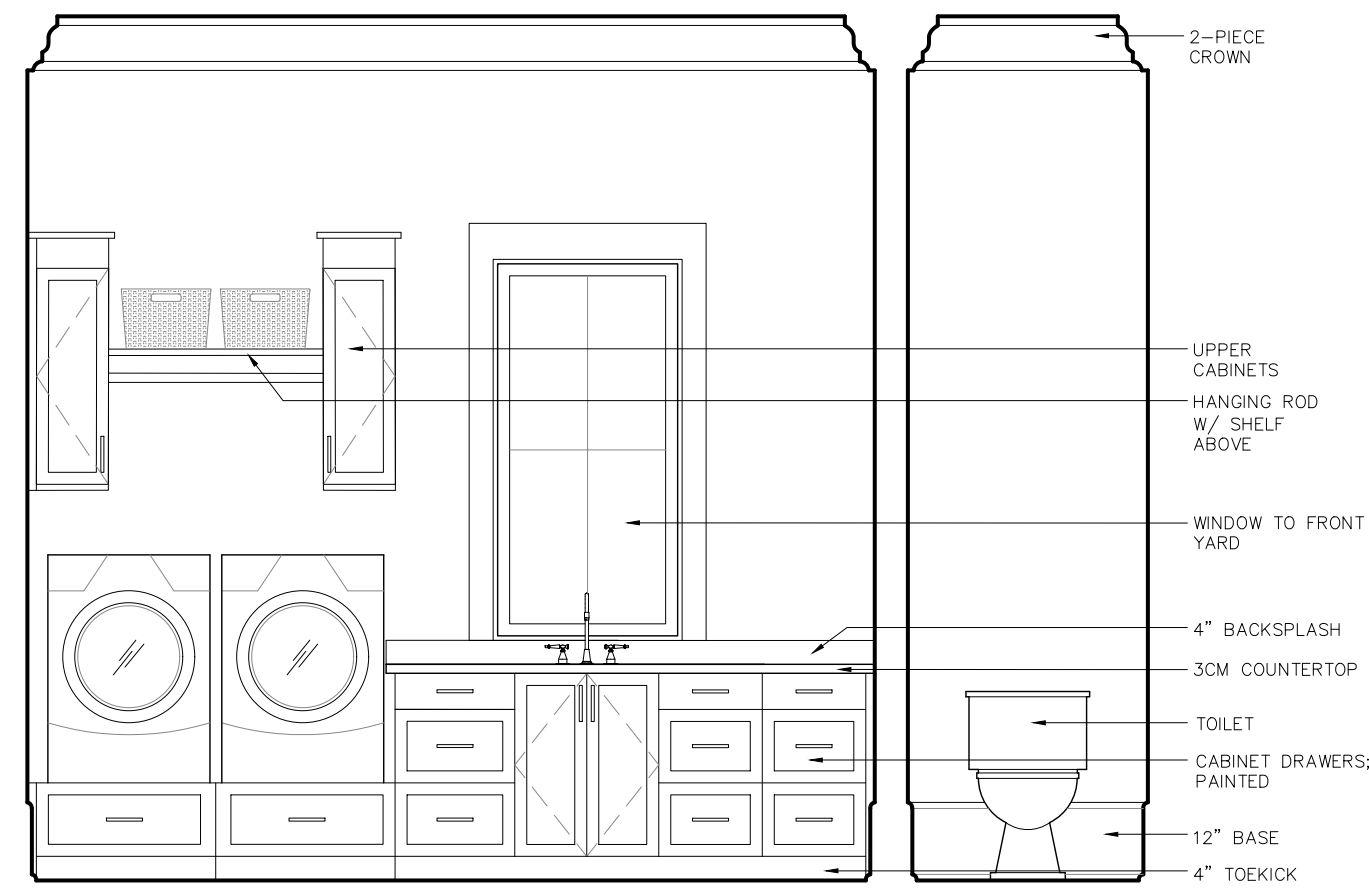
2 Utility Scale: 3/8" = 1'-0"
