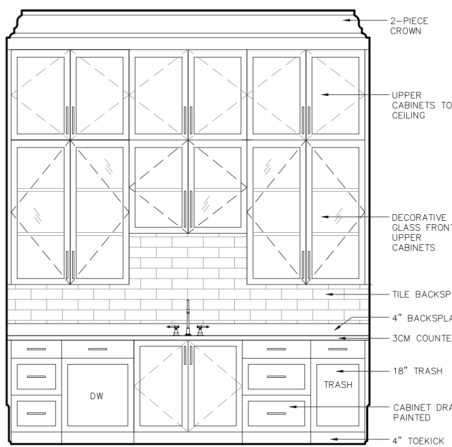
5 Dirty Kitchen Scale: 3/8" = 1'-0"
