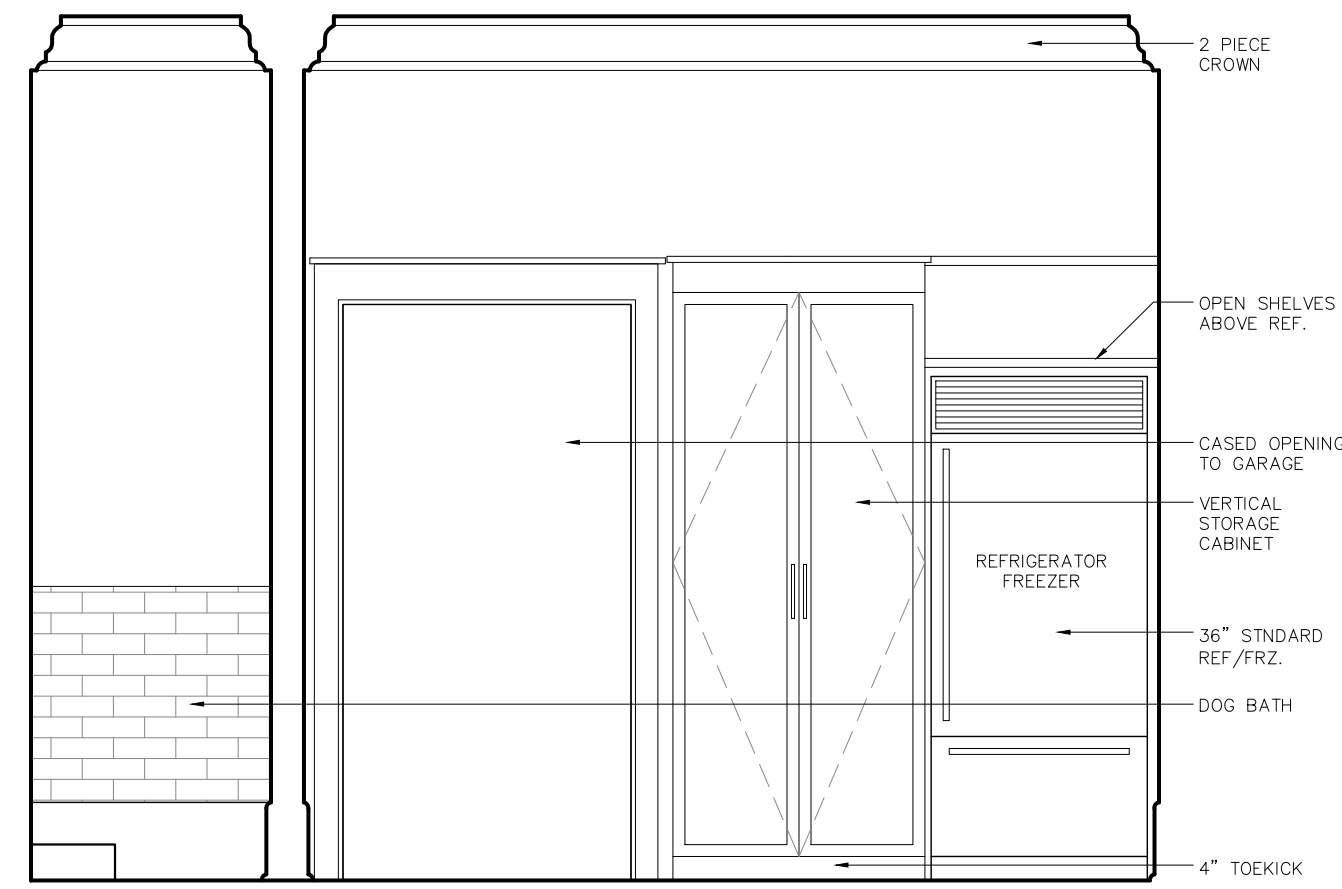
1 Utility Scale: 3/8" = 1'-0"
