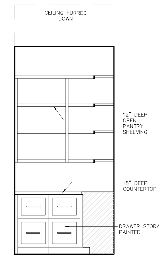
7 Pantry Scale: 3/8" = 1'-0"
