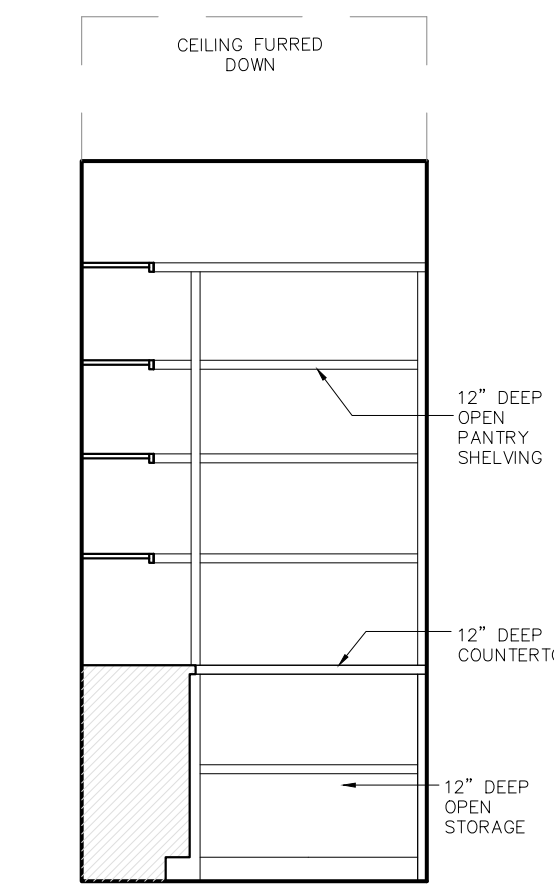
9 Pantry Scale: 3/8" = 1'-0"
