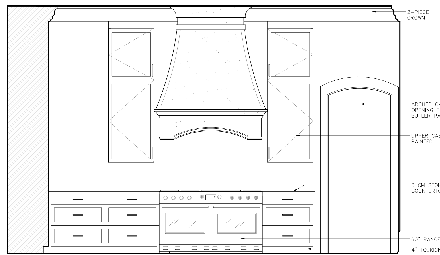
12 Kitchen Scale: 3/8" = 1'-0"
