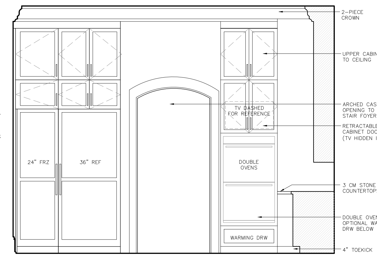
13 Kitchen Scale: 3/8" = 1'-0"
