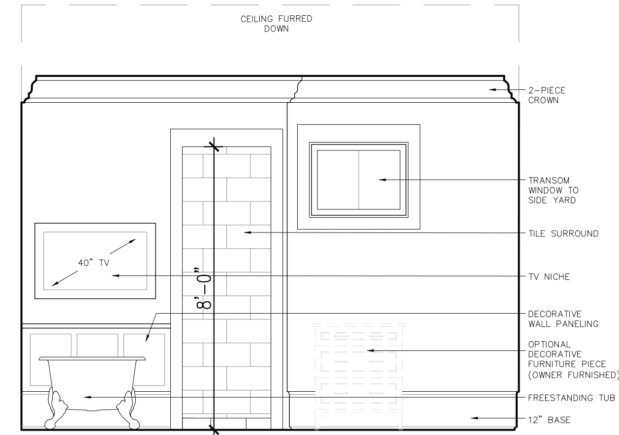
4 Master Bath Scale: 3/8" = 1'-0"
