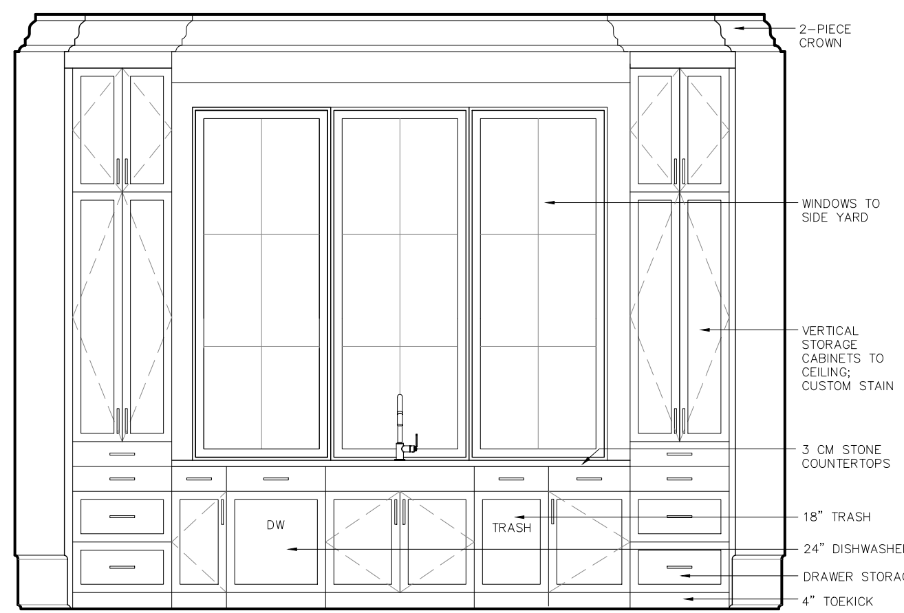
11 Kitchen Scale: 3/8" = 1'-0"
