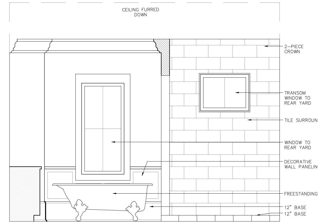
3 Master Bath Scale: 3/8" = 1'-0"
