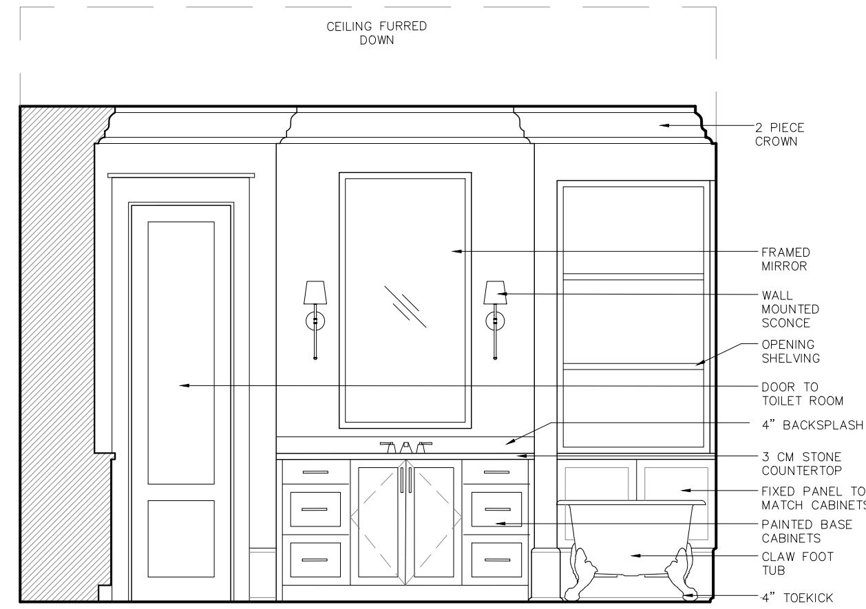
2 Master Bath Scale: 3/8" = 1'-0"
