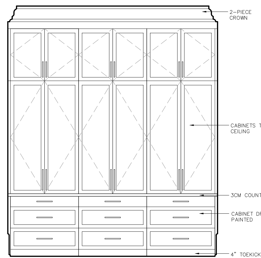
6 Dirty Kitchen Scale: 3/8" = 1'-0"
