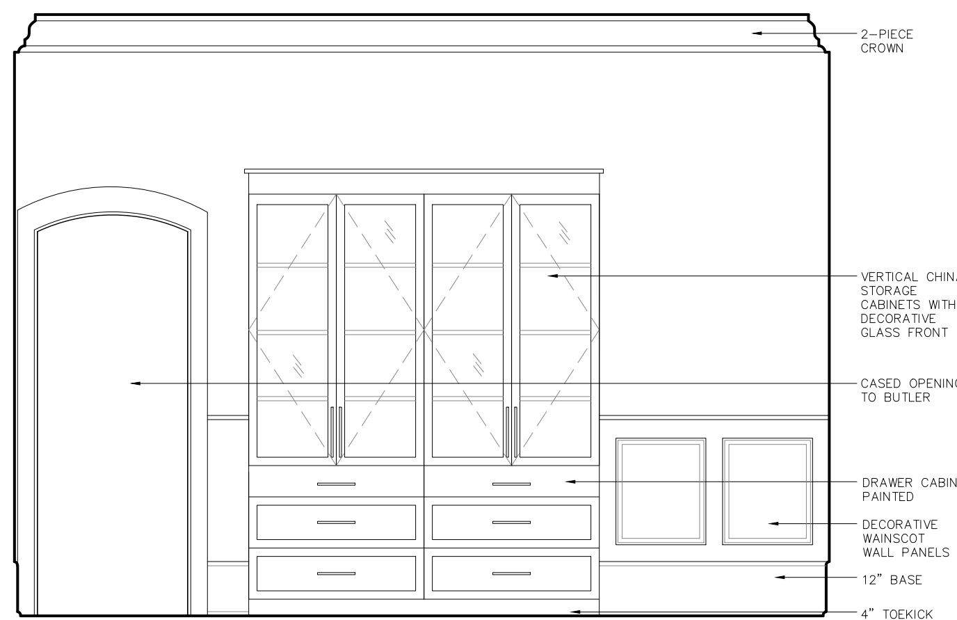
10 Dining Scale: 3/8" = 1'-0"
