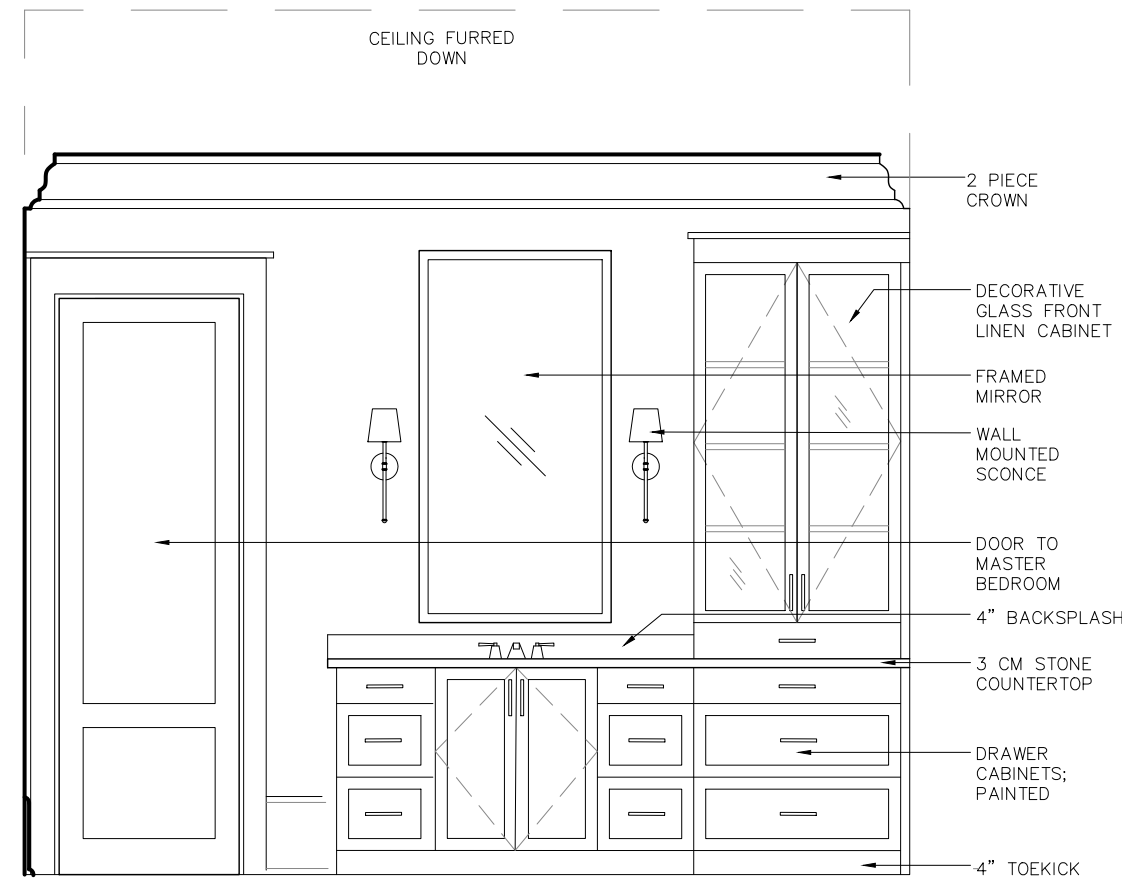
1 Master Bath Scale: 3/8" = 1'-0"
