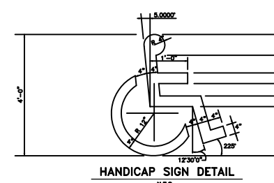
HANDICAP SIGN DETAIL N.T.S.
