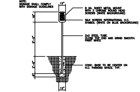
EXTERIOR HANDICAP SIGN N.T.S.
