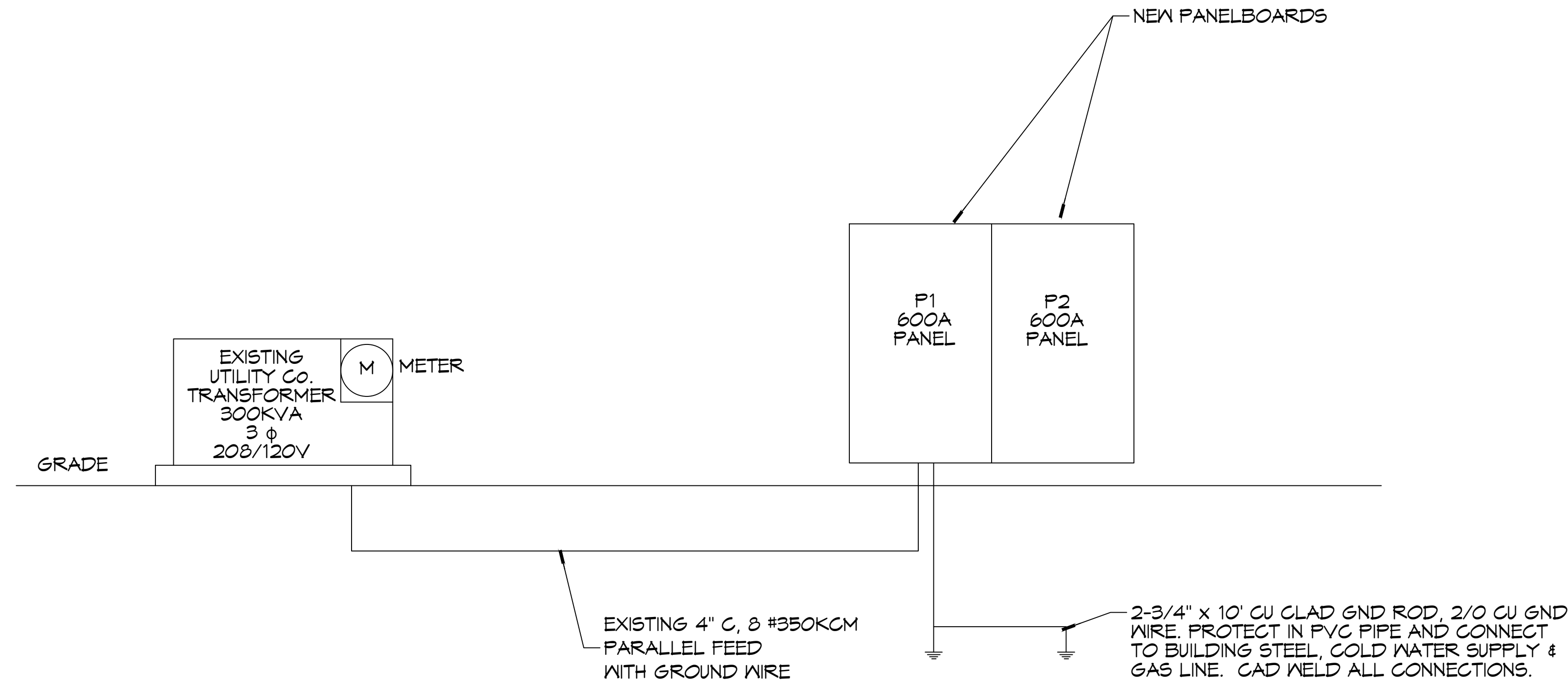
RISER DIAGRAM SCALE: NTS
