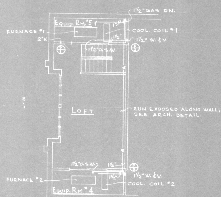
LOFT PLAN SCALE: 1/8" = 1'-0"
