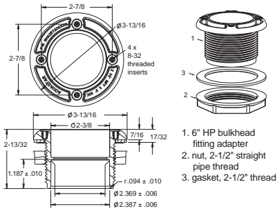
Part # 6E15Txxx
