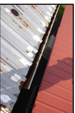
CORRODED GUTTERS N.T.S.
