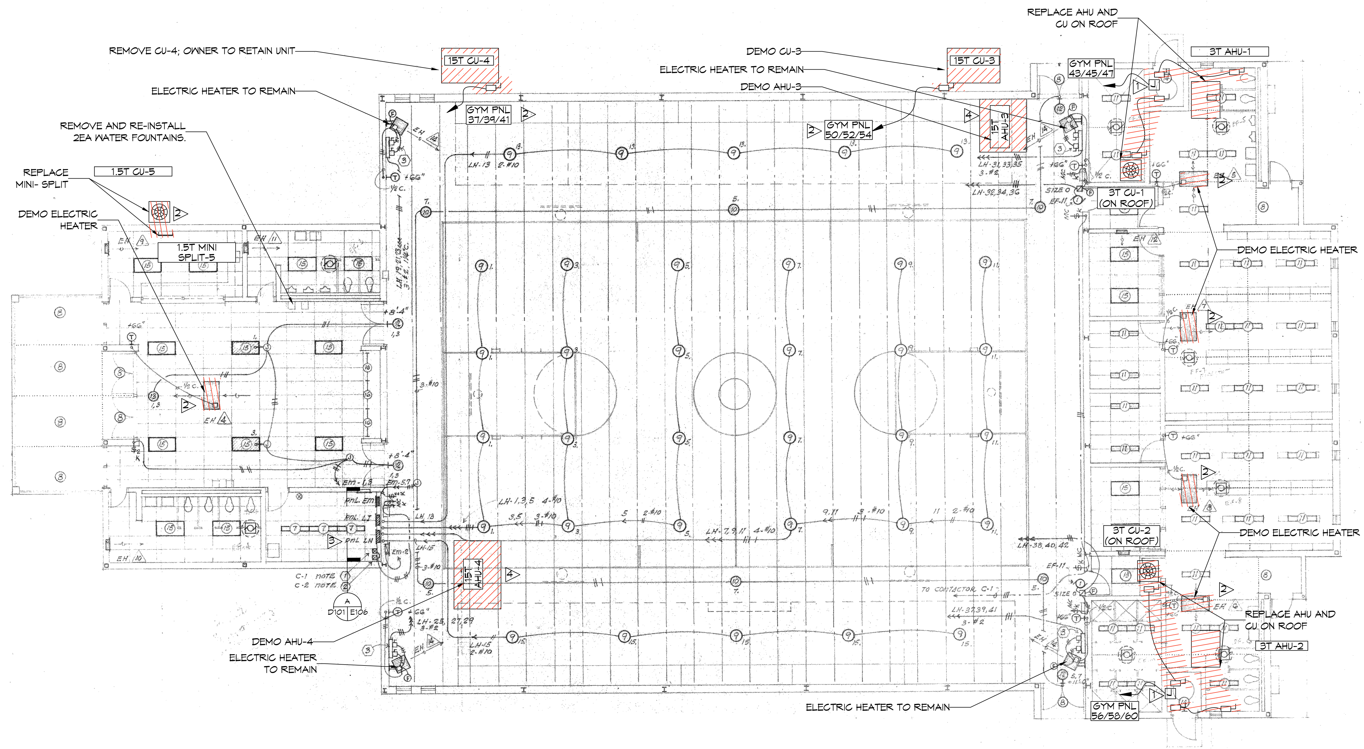
1 DEMO PLAN SCALE: 1/8" = 1'-0"
