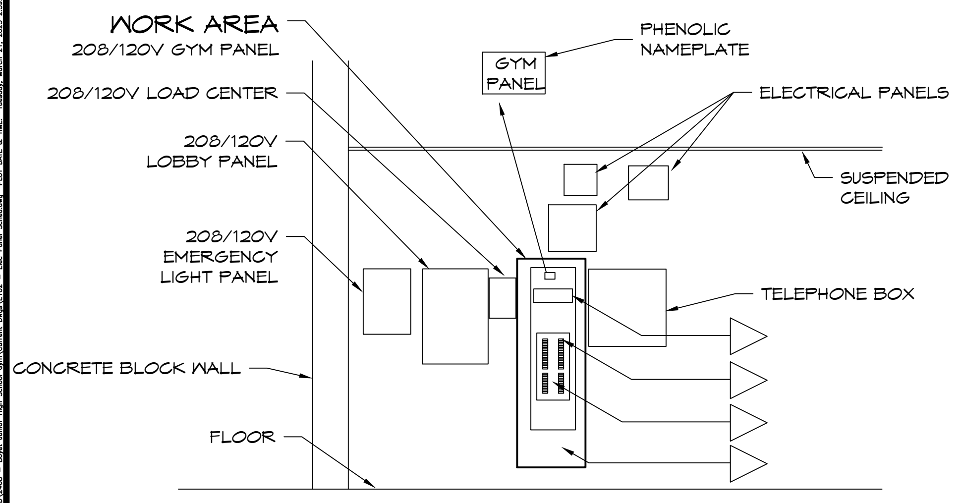
H ELEVATION E101 E102 SCALE: NONE
