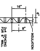
WALL DETAIL SCALE: 1/4" = 1'-0" A-10
