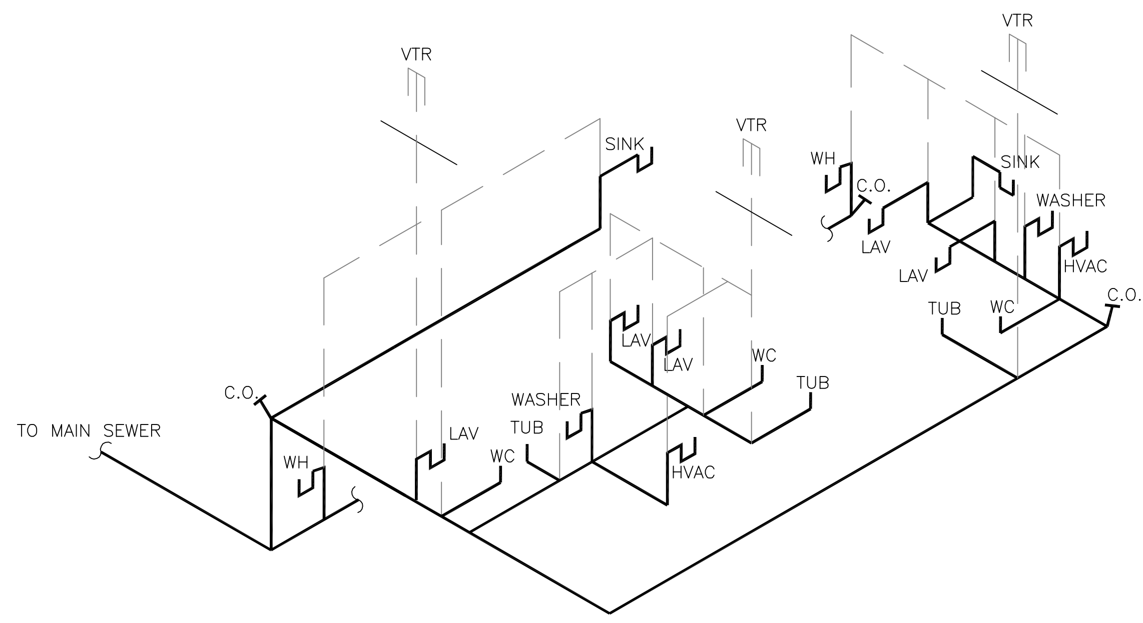
RISER DIAGRAM N.T.S.
