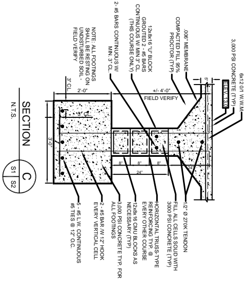
SECTION B S1 S2 N.T.S.
