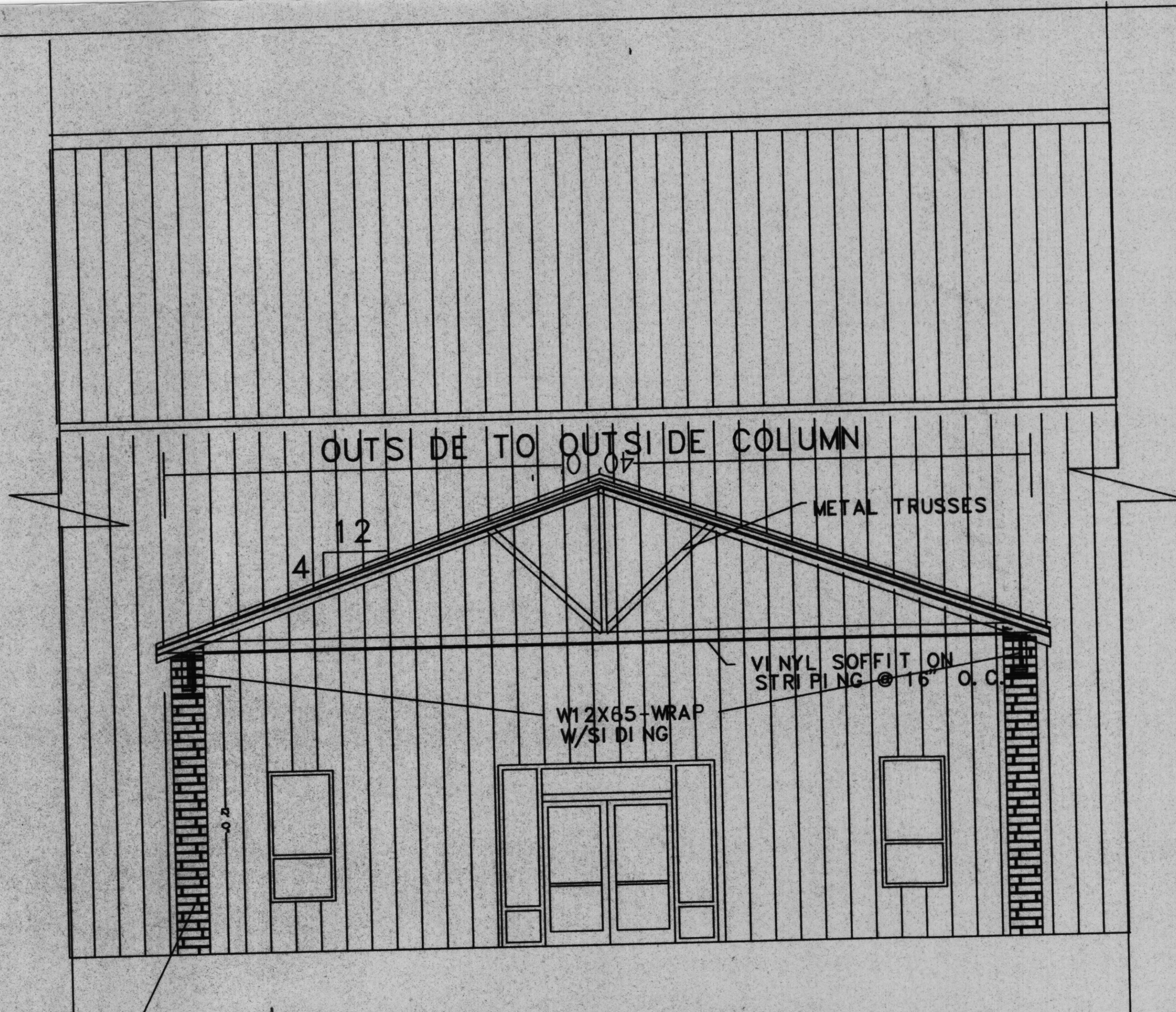
END ELEVATION
