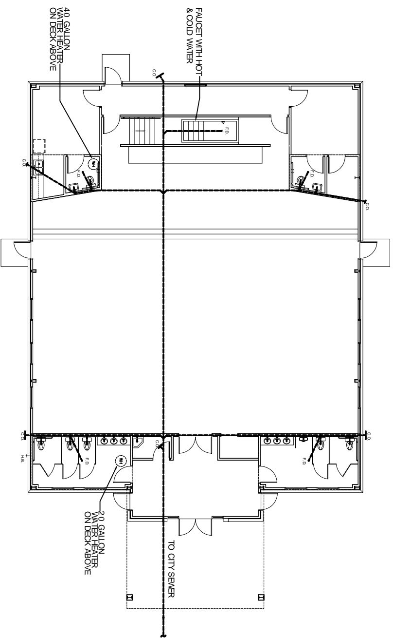
PLUMBING PLAN SCALE: 1/8" = 1'
