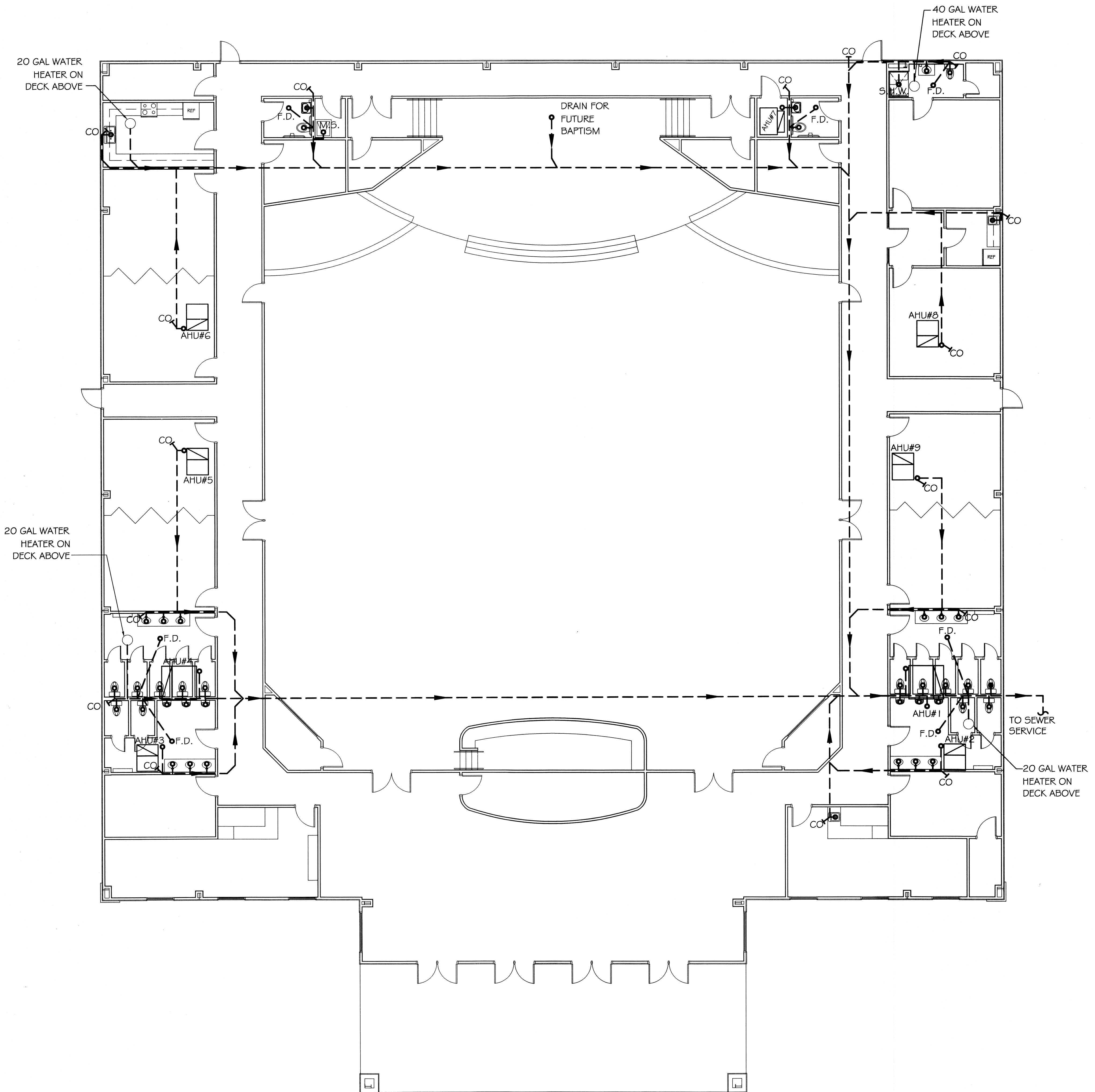
PLUMBING PLAN SCALE: 1/8" = 1'-0"
