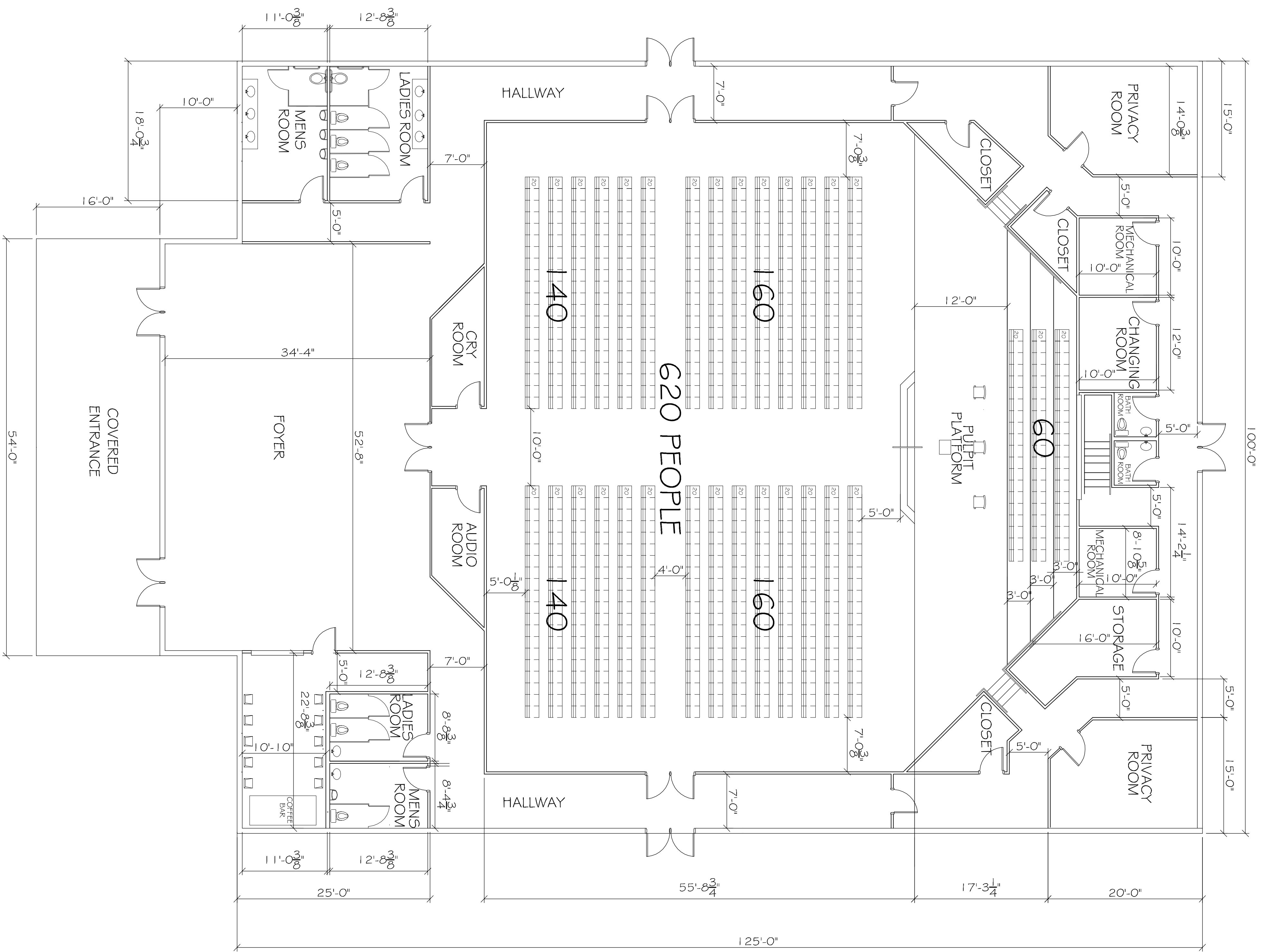
FLOOR PLAN SCALE: 1/8" = 1'
