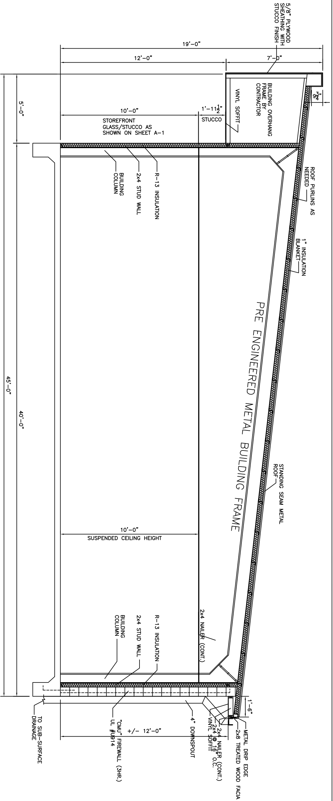
A CROSS SECTION SCALE: 1/2" = 1'-0"
