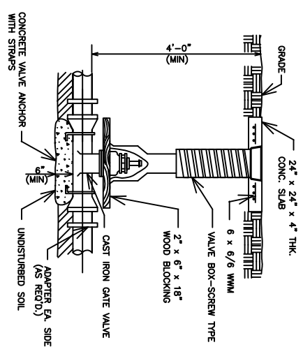
TYPICAL VALVE BOX DETAIL SCALE: N.T.S.
