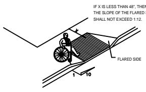
FIG. 13 BUILT-UP CURB RAMP N.T.S.
