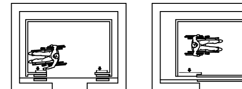
FIG. 23 CAR CONTROLS N.T.S.
