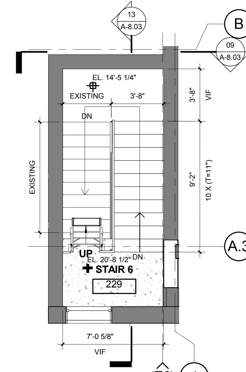
STAIR-6 LOGE LEVEL
