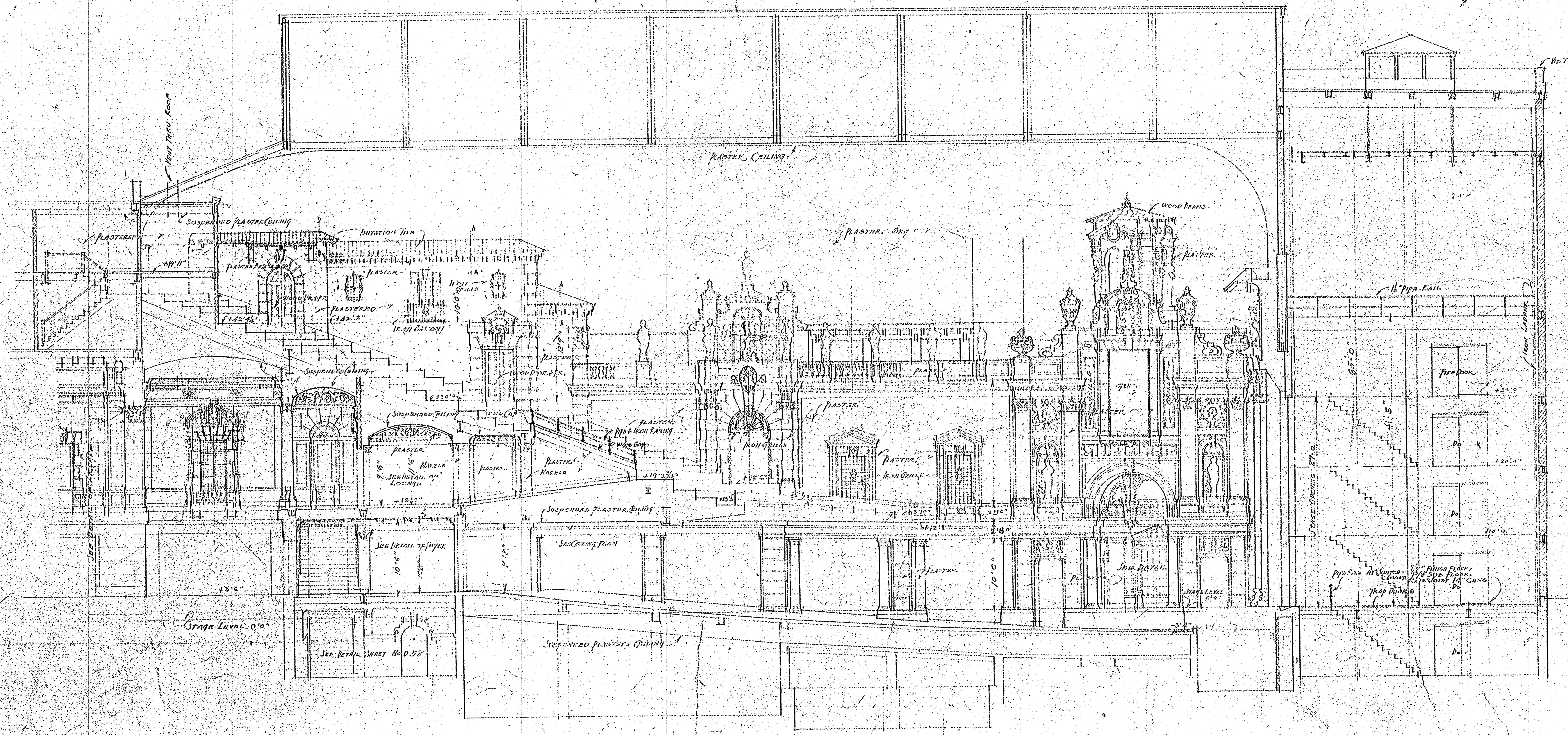
LONGITUDINAL SECTION LOOKING TOWARD N. SARATOGA ST. SCALE 1/8" = 1'-0"
