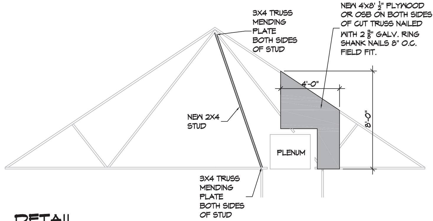
DETAIL SCALE: N.T.S.
