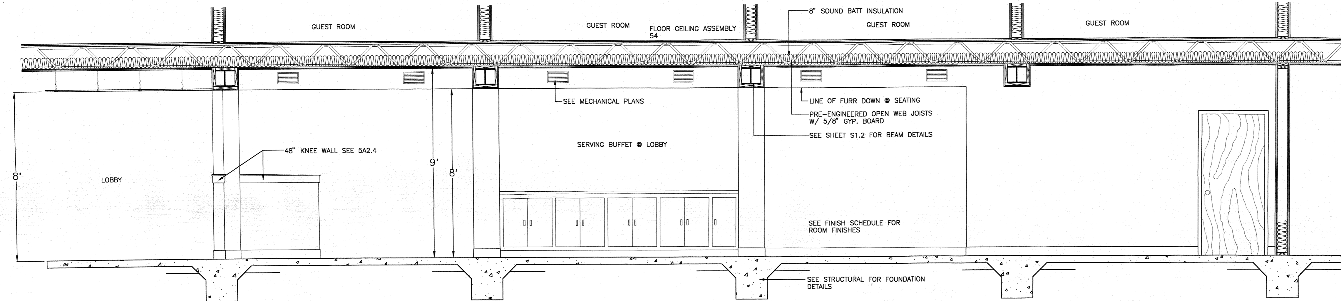
7 SECTION THRU LOBBY SCALE: 3/8" = 1'-0"
