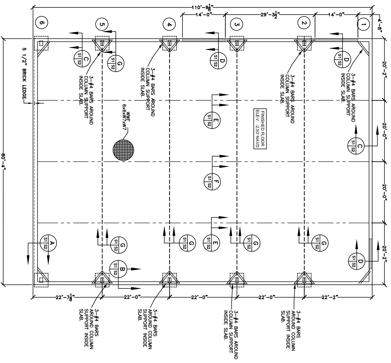
FOUNDATION SCALE: 1/8"=1'-0"
