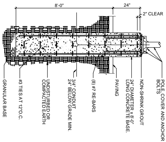
LIGHT POLE DETAIL N.T.S.
