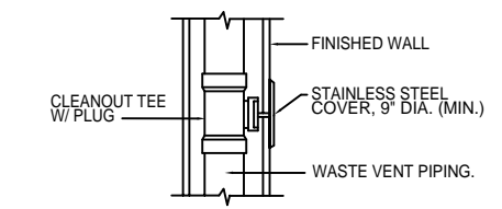
WALL CLEANOUT DETAIL N.T.S.
