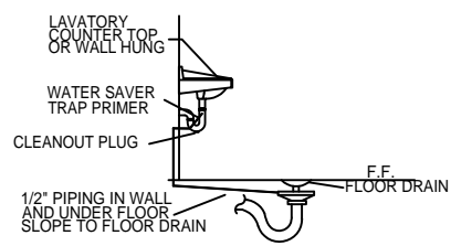
FLOOR DRAIN DETAIL N.T.S.
