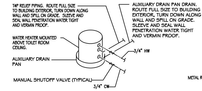
WATER HEATER DETAIL N.T.S.
