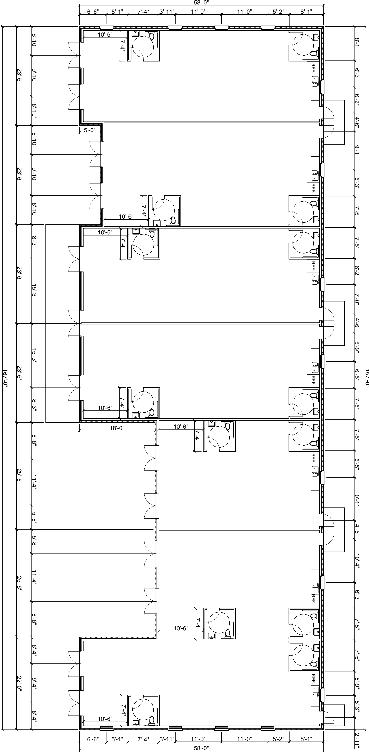
FLOOR PLAN SCALE: 1/8" = 1'-0"
